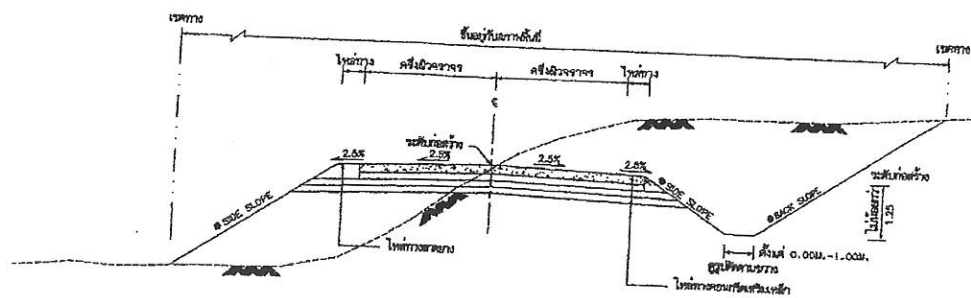
รูปตัดตามขวางแสดงด้านคันและสันดิน
