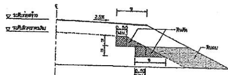
รูปตัดขวางของคันทางและคันดิน
