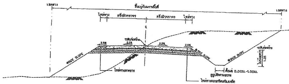
รูปตัดขวางของคันทางและคันดิน
