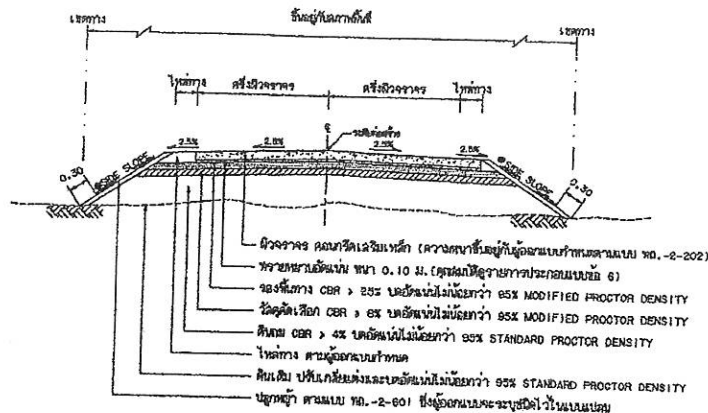
รูปตัดขวางของคันทางและคันดิน
