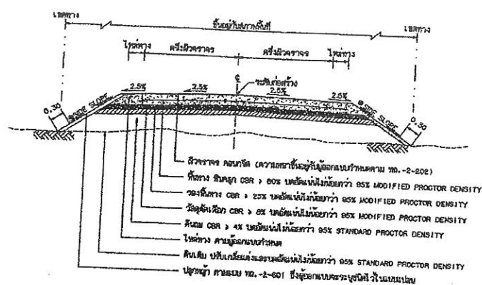
รูปตัดแสดงโครงสร้างถนนคอนกรีตเสริมเหล็กและคูระบายน้ำ
