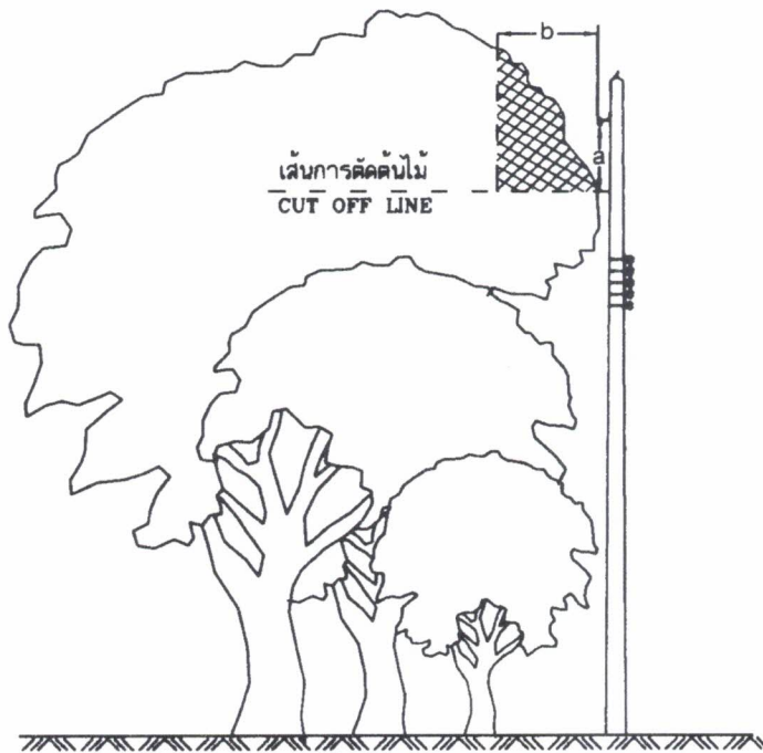
การตัดแต่งต้นไม้สำหรับสายหุ้มฉนวนเต็มพิกัดดีเกลือ TREE TRIMMING FOR TWISTED AERIAL CABLE.
