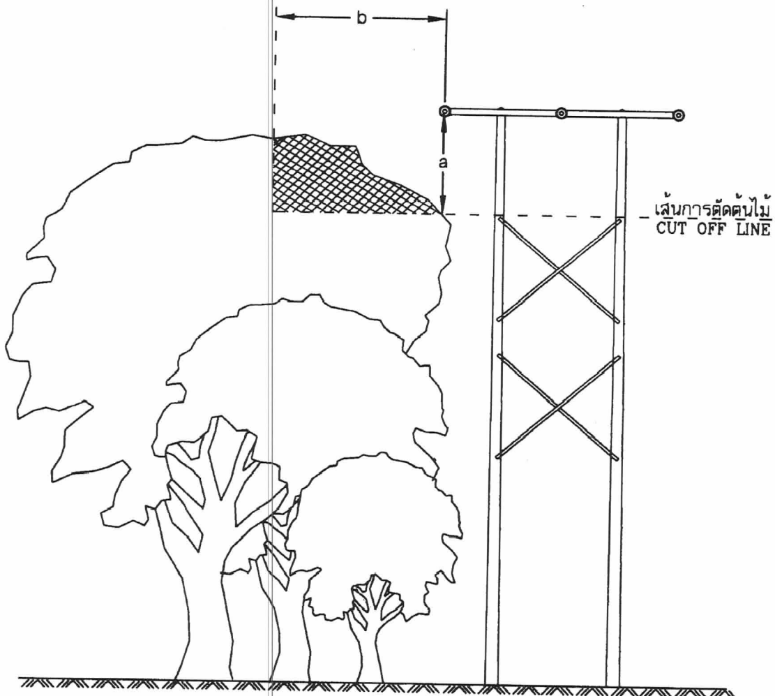
การตัดแต่งต้นไม้สำหรับสายเปลือยแรงสูงที่มีระยะทางระหว่างเสาตั้งแต่ 100 เมตร ขึ้นไป TREE TRIMMING FOR H.V. BARE CONDUCTOR WITH SPANS OF 100 m AND ABOVE.
