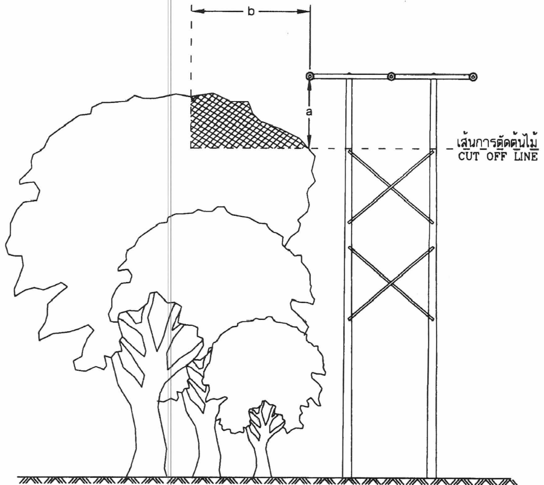
การตัดแต่งต้นไม้สำหรับสายเปลือยแรงสูงที่มีระยะห่างระหว่างเสาตั้งแต่ 100 เมตร ขึ้นไป TREE TRIMMING FOR H.V. BARE CONDUCTOR WITH SPANS OF 100 m AND ABOVE.
