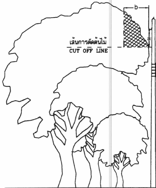
การตัดแต่งต้นไม้สำหรับสายหุ้มฉนวนเต็มพิกัดเกลียว TREE TRIMMING FOR TWISTED AERIAL CABLE.
