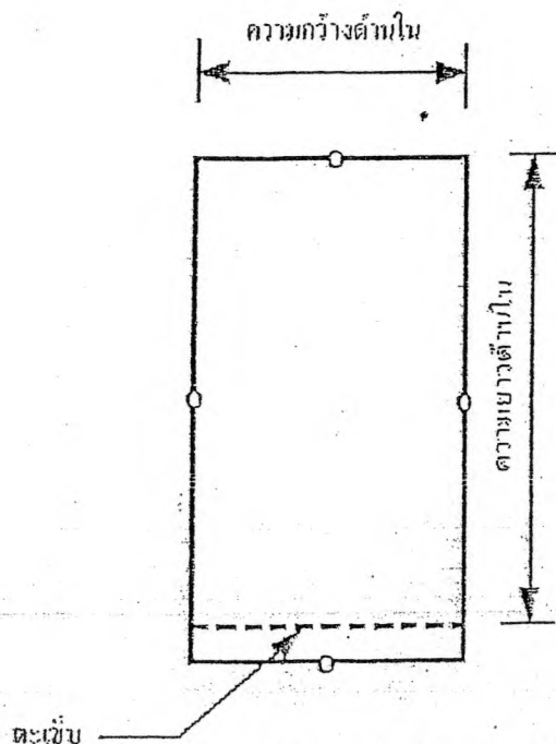
รูปที่ 1 กระสอบแบบธรรมดา (ข้อ 3.2.1 และข้อ 10.2.2.1)
