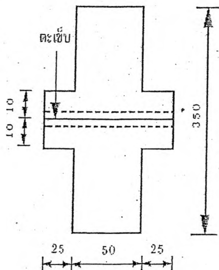
รูปที่ 3 รูปร่างและขนาดของชิ้นทดสอบสำหรับทดสอบ แรงดึงสูงสุดของตะเข็บกันกระสอบ (ข้อ 10.6.2)
