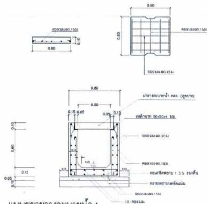
แบบขยายรางระบายน้ำ 1
