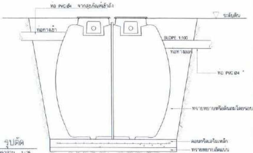
แบบขยายถังบำบัดน้ำเสียสำเร็จรูป
