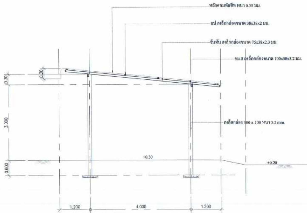
รูปตัด มาตราส่วน 1:50
