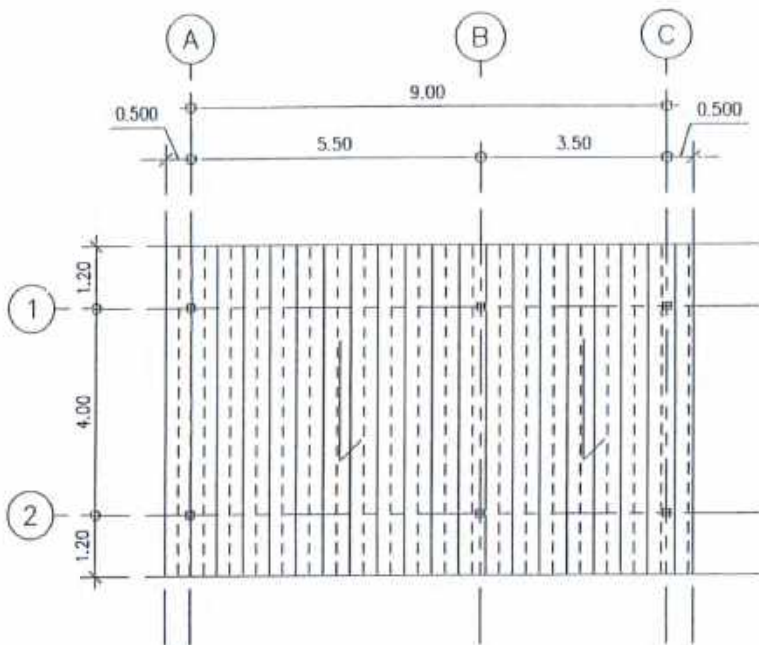
แปลนหลังคาโรงจอดรถ
