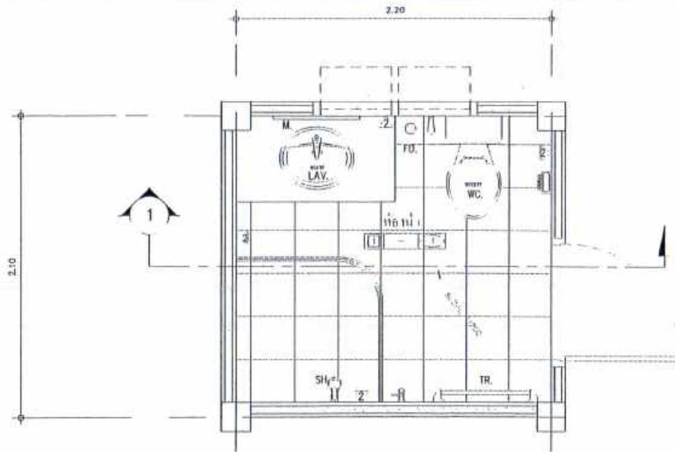
แปลนห้องน้ำ (WC.) มาตราส่วน 1 : 25
