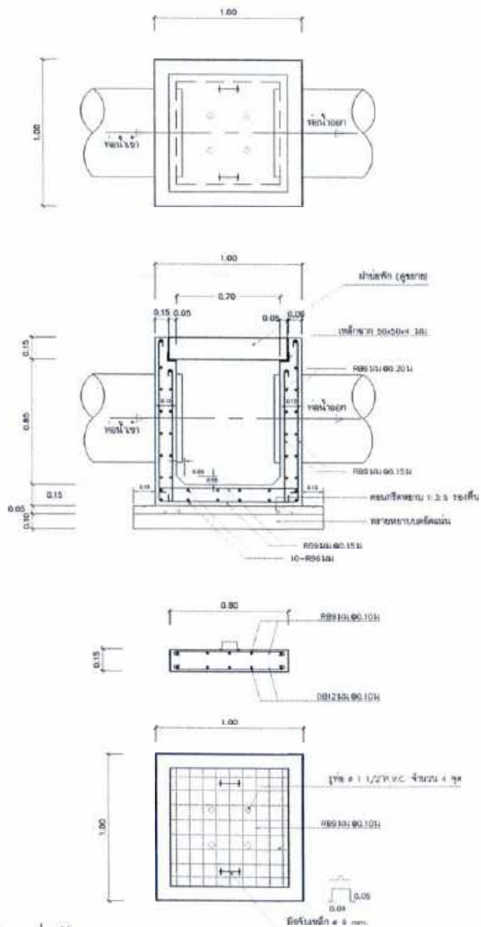
แบบขยายบ่อพัก
