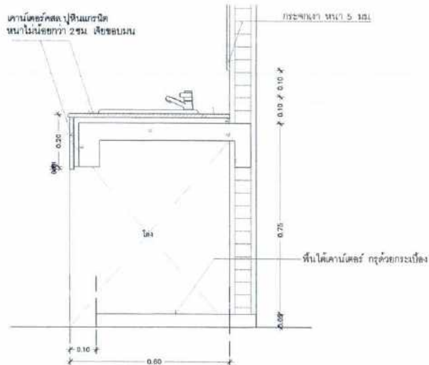
แบบขยายครานเตอร์อ่างล้างมือ มาตราส่วน 1 : 10
