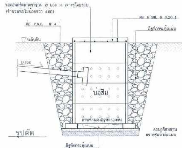
แบบขยายบ่อซีเมนต์น้ำทิ้ง
