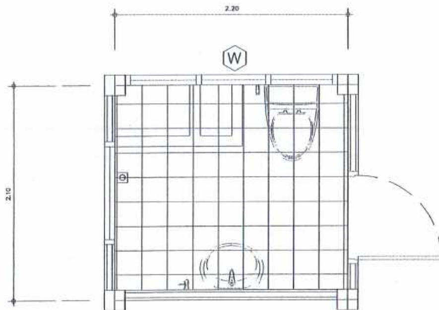
แปลนห้องน้ำ (เดิม) มาตราส่วน 1 : 25
