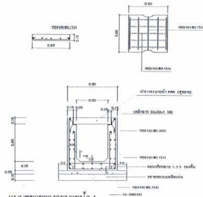
แบบขยายรางระบายน้ำ 1 มาตราส่วน 1 : 25
