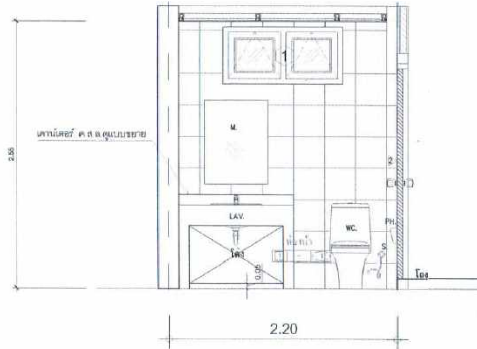
รูปตัดห้องน้ำ (WC.) มาตราส่วน 1 : 25
