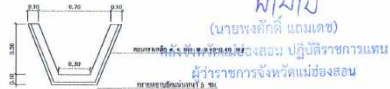
แบบขยายรางระบายน้ำ 2 มาตราส่วน 1 : 25
