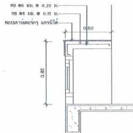
แบบขยายรูปตัดเคาน์เตอร์ มาตราส่วน 1:25
