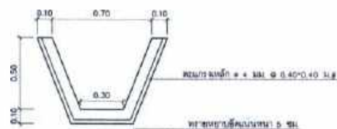
แบบขยายรางระบายน้ำ 2
