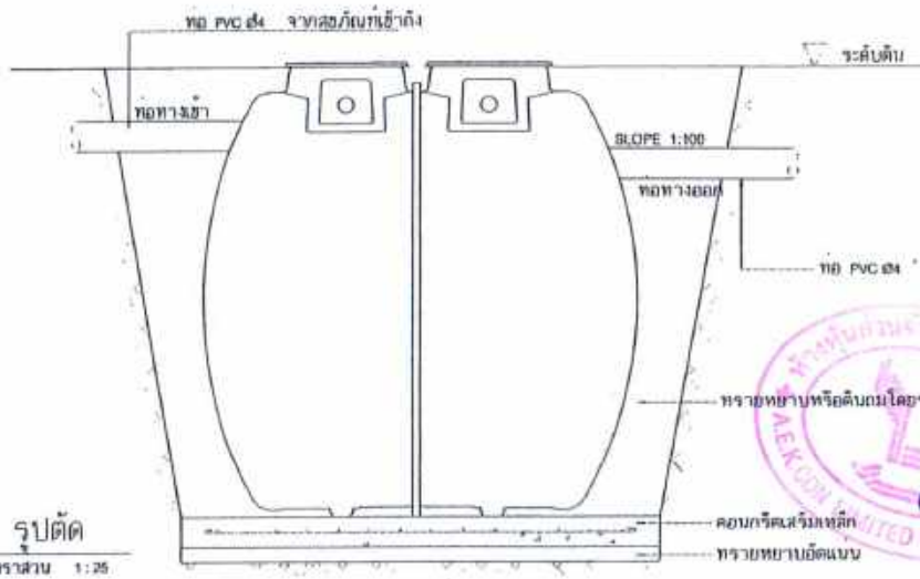
แบบขยายถังบำบัดน้ำเสียสำเร็จรูป มาตราส่วน 1:25
