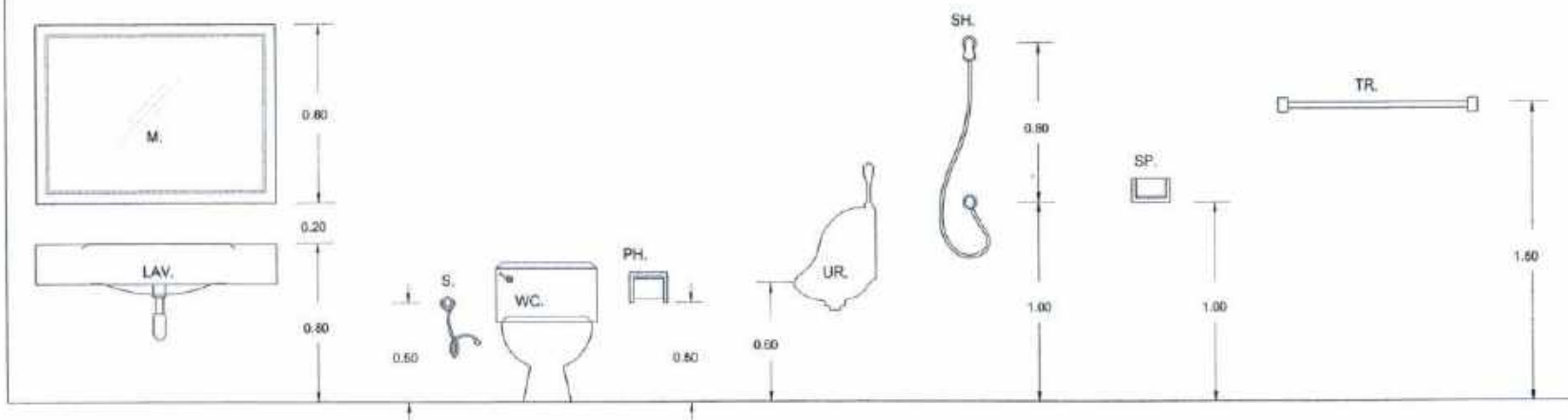
มาตรฐานการติดตั้งสุขภัณฑ์
