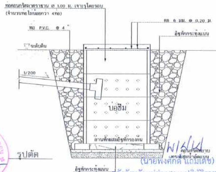
แบบขยายบ่อซึมน้ำทิ้ง มาตราส่วน 1:25
