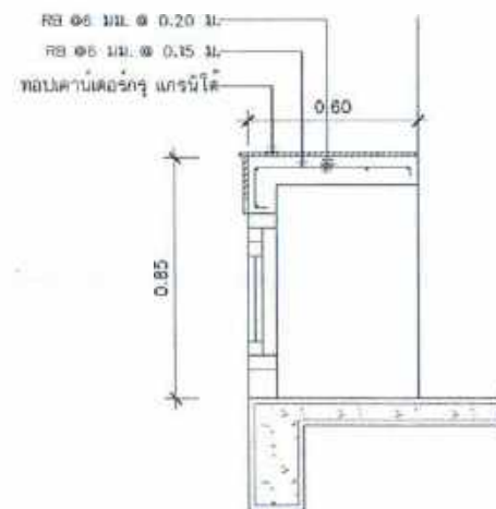
แบบขยายรูปตัดเคาน์เตอร์ มาตราส่วน 1:25
