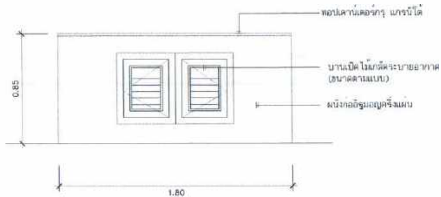
แบบขยายรูปเคาน์เตอร์ มาตราส่วน 1:25
