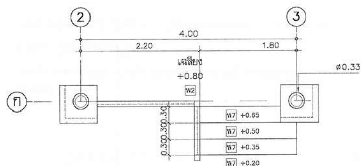
แปลนขยายระบียงชั้นล่าง
