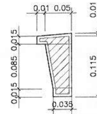
แบบขยายบัวหัวเสาทั่วไป มาตราส่วน 1:5
