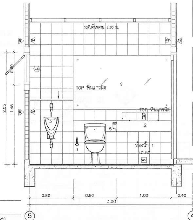
รูปตัดขยายห้องน้ำ ก มาตราส่วน 1:25
