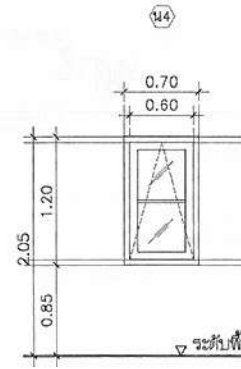
หน้าต่างบานกระทุ้ง วงกบอลูมิเนียม วงกบอลูมิเนียม ลูกฟักกระจากสีหนา 5 มม.
