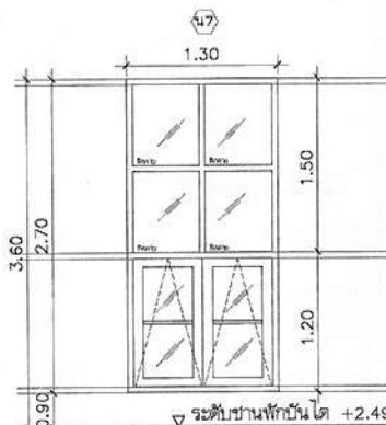
หน้าต่างบานกระทุ้ง พร้อมบานติดตาย วงกบอลูมิเนียม กรอบบานอลูมิเนียม ลูกฟักกระจากสีขาวสีหนา 5 มม.
