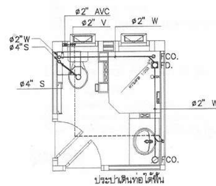
แปลนห้องน้ำทิ้งห้องน้ำ 3 มาตราส่วน 1:25
