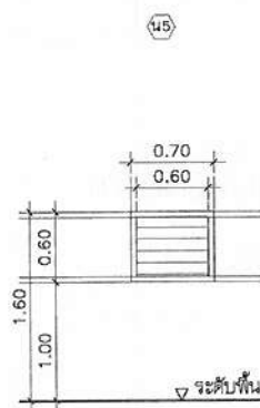
หน้าต่างบานกระปับนวม วงกบอลูมิเนียม ลูกฟักกระจากสีขาวสีหนา 5 มม. ลูกฟักขนาดกว้าง 4 1/2" สมนวม
