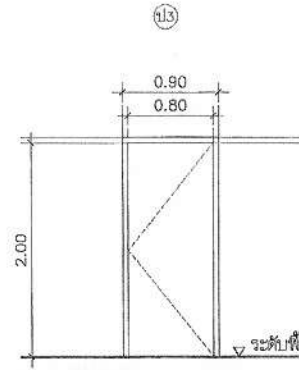
ประตูบานเปิดเดี่ยวลวดลายรูป วงกบไม้สัก ขนาด 2"x4" ทาสีน้ำมัน 2 ด้าน ผลิตกันท่อนของ DORIC รุ่นคลาสสิก หรือเทียบเท่า
