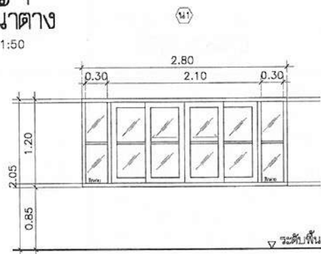
หน้าต่างบานเลื่อนคู่ พร้อมบานกระจัดตาย วงกบอลูมิเนียม วงกบอลูมิเนียม ลูกฟักกระจากสีหนา 5 มม.
