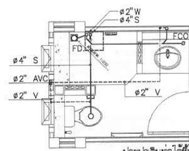
แปลนห้องน้ำทิ้งห้องน้ำ 2 มาตราส่วน 1:25
