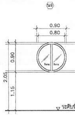
หน้าต่างบานกระจัดตาย วงกบไม้สักขนาด 2"x4" ลูกฟักกระจากสีหนา 5 มม./ไม้สักเข้าลิ้น
