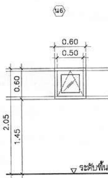
หน้าต่างบานกระทุ้ง วงกบอลูมิเนียม ลูกฟักกระจากสีขาวสีหนา 5 มม.
