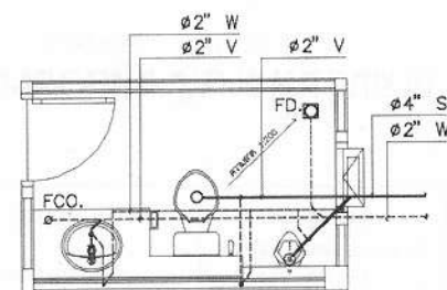
แปลนห้องน้ำทิ้งห้องน้ำ 1 มาตราส่วน 1:25
