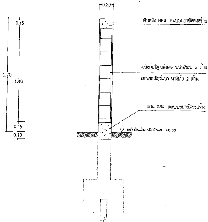
รูปตัดขยายรั้ว มาตราส่วน 1:50
