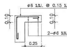
แบบขยายปีกนกค.ส.ล. มาตราส่วน 1:25
