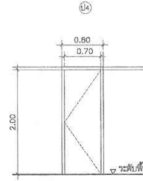
ประตูบานเปิดเดี่ยว วงกบไม้สัก ขนาด 2"x4" กรอบบานไม้สักดัดกันน้ำ ทาสีน้ำมัน 2 ด้าน
