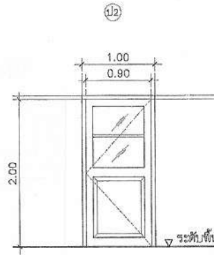
ประตูบานเปิดเดี่ยว วงกบไม้สัก ขนาด 2"x4" กรอบบานไม้สัก 1 1/2" x 4" ลูกฟักไม้สัก 3/4"x4" เข้าเส้น ทาสีน้ำมัน 1 ด้าน ย้อมสี 1 ด้าน
