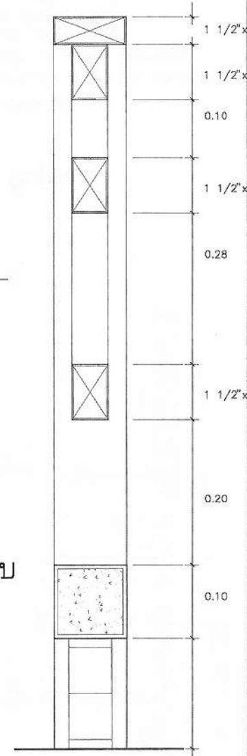
แบบขยาย ก มาตราส่วน 1:5
