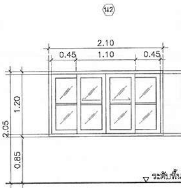
หน้าต่างบานเลื่อนคู่ วงกบอลูมิเนียม วงกบอลูมิเนียม ลูกฟักกระจากสีหนา 5 มม.
