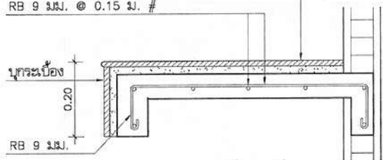
แบบขยายเคาน์เตอร์ คสล. มาตราส่วน 1:10
