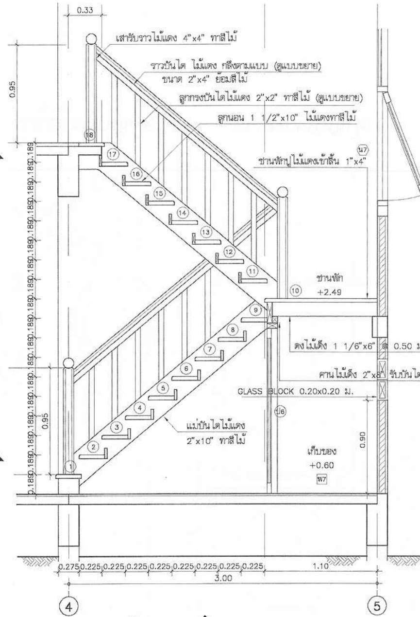
รูปตัดบันได ก
