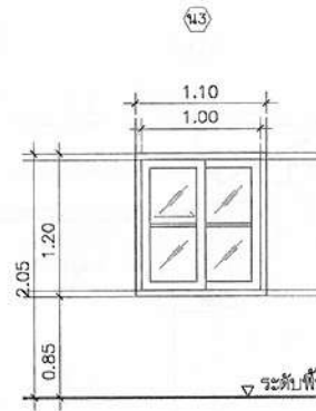
หน้าต่างบานเลื่อน วงกบอลูมิเนียม วงกบอลูมิเนียม ลูกฟักกระจากสีหนา 5 มม.
