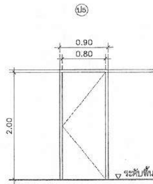
ประตูบานเปิดเดี่ยว วงกบไม้สัก ขนาด 2"x4" กรอบบานไม้สักดัดกันน้ำ ทาสีน้ำมัน 2 ด้าน
