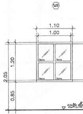
หน้าต่างบานกระจัดตาย วงกบอลูมิเนียม ลูกฟักกระจากสีหนา 5 มม.
