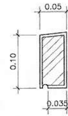
แบบขยายหลังวงกบ มาตราส่วน 1:5
