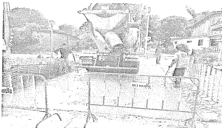
ภาพถ่ายงานซ่อมแซมถนนคอนกรีต ซอยสี่ตา
