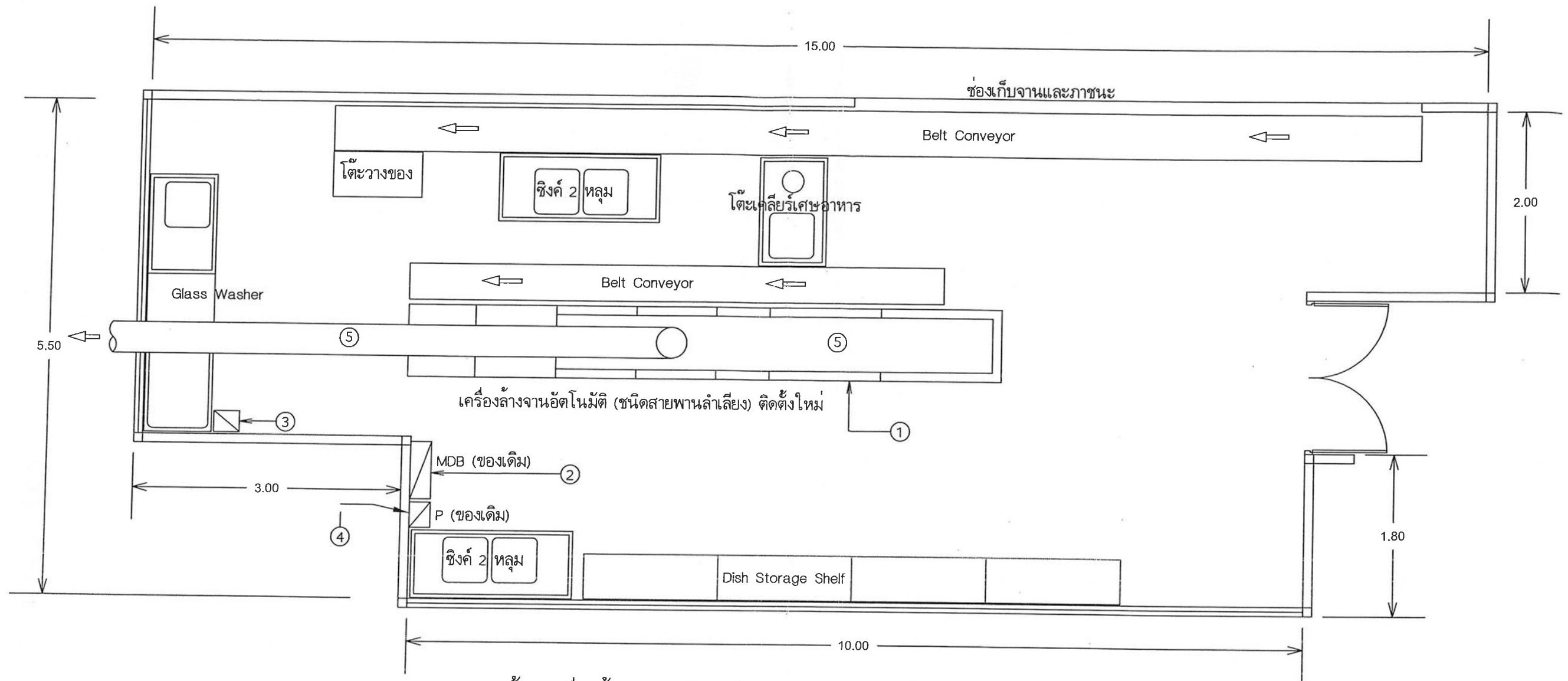
แปลนห้องเครื่องล้างจาน (โซนบี) (แสดงการติดตั้งเครื่องล้างจานโซนบี) มาตรฐาน 1 : 50
