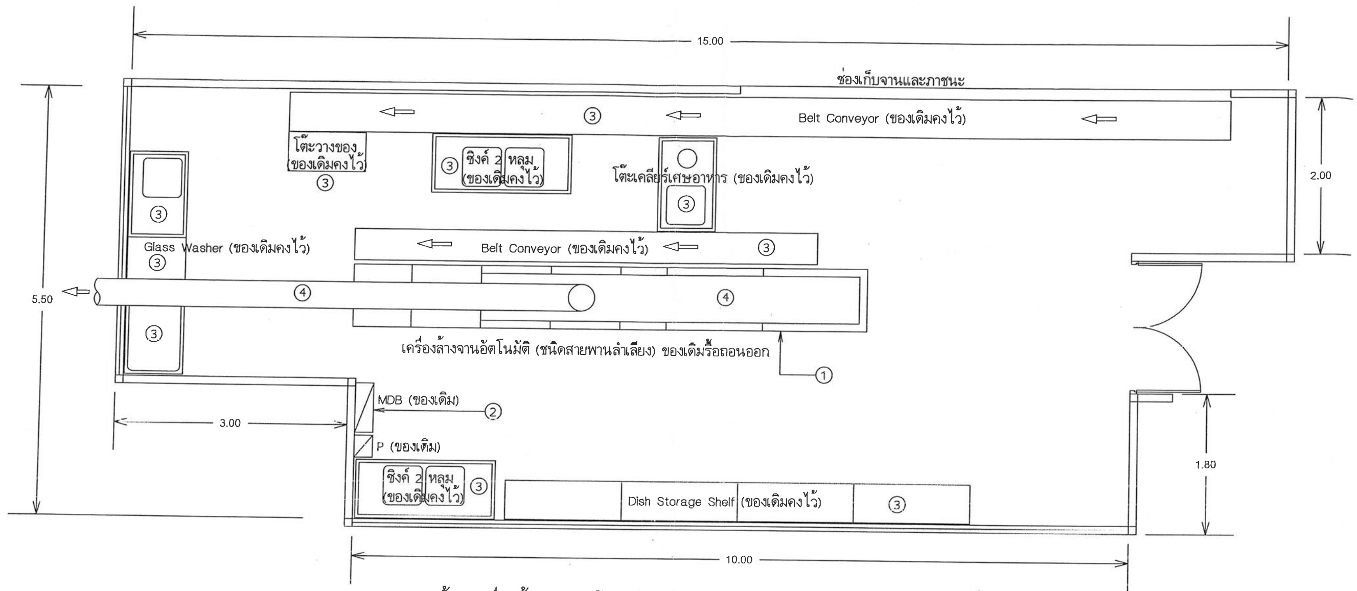
แปลนห้องเครื่องล้างจาน (โซนบี) (แสดงการรื้อถอนเครื่องล้างจานโซนบี) มาตรฐาน 1 : 50
