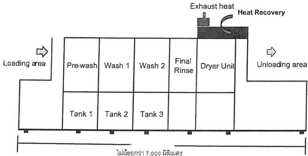
รูปที่ 1 แสดงลักษณะการทำงานของเครื่องล้างจานอัตโนมัติ (ชนิดสายพานลำเลียง)
