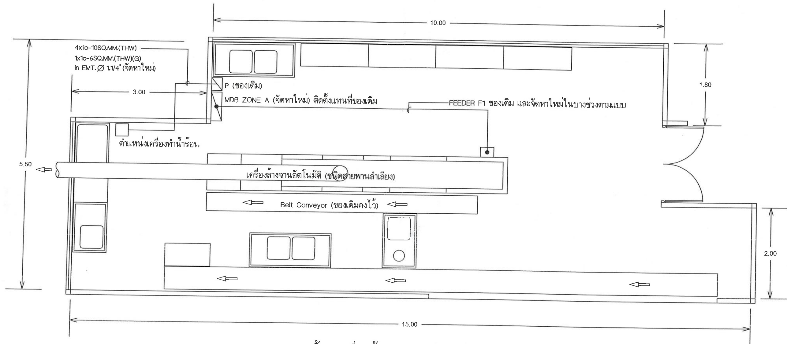
แปลนห้องเครื่องล่างงาน (ZONE A)
