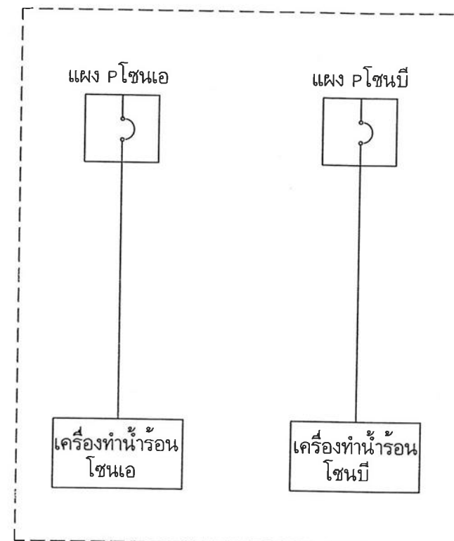
SINGLE LINE DIAGRAM FOR เครื่องทำน้ำร้อนติดตั้งใหม่
