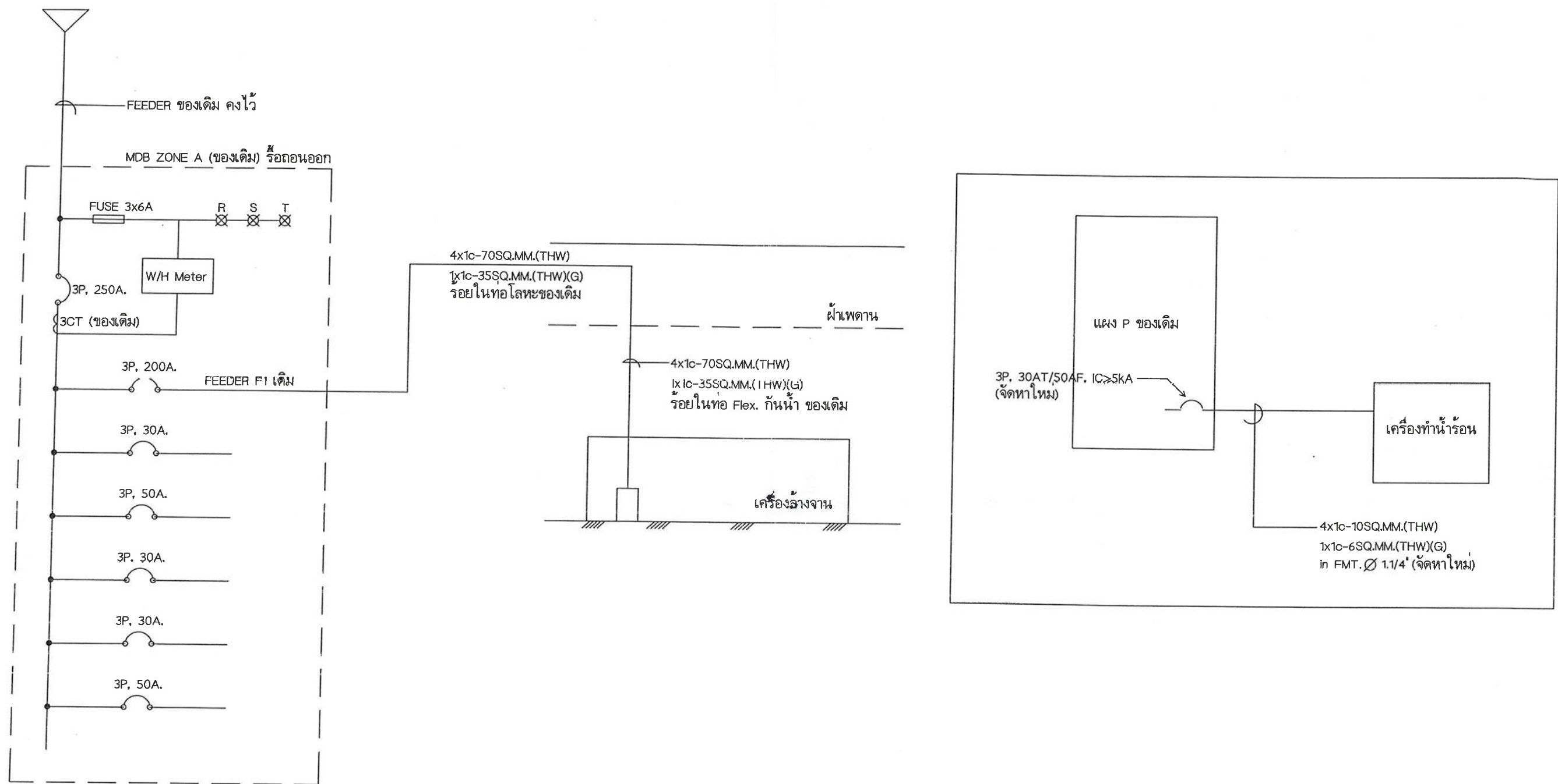
ระบบไฟฟ้าห้องเครื่องล้างจานด้านทิศเหนือ (ZONE A) ของเดิม ก่อนปรับปรุง
