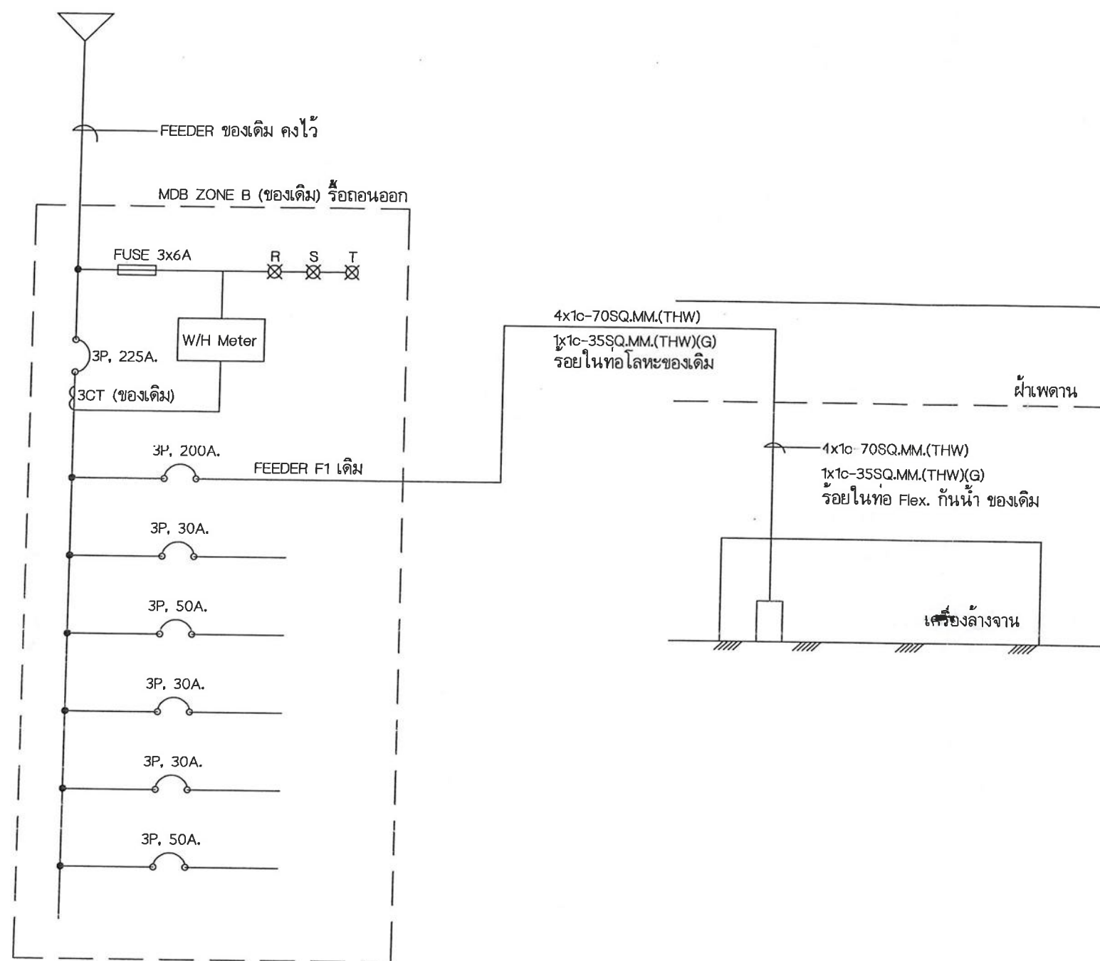
ระบบไฟฟ้าห้องเครื่องล้างจานด้านทิศใต้ (ZONE B) ของเดิม ก่อนปรับปรุง
