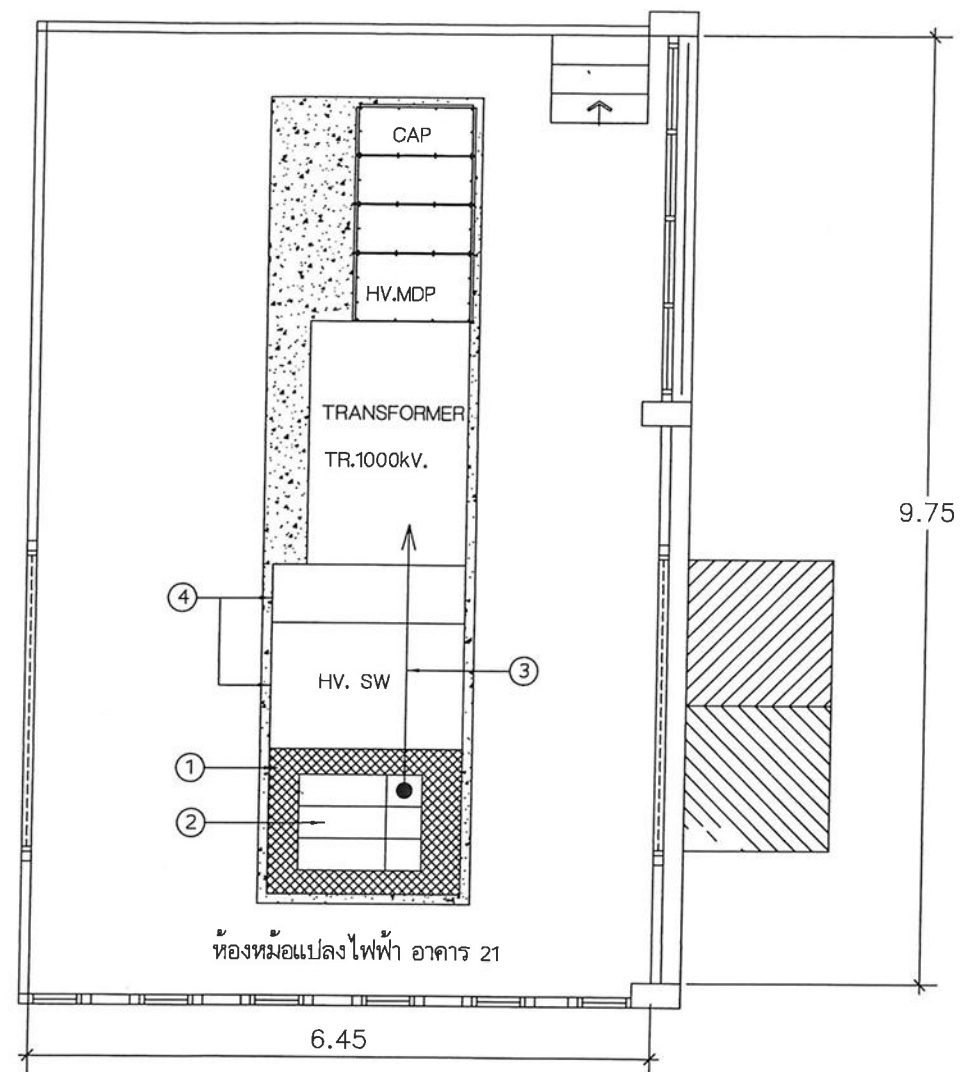
แบบแสดงตำแหน่งตู้ RMU. ที่เปลี่ยนแทนตู้ HV. Switch ของเดิม หน่วยเป็น เมตร
