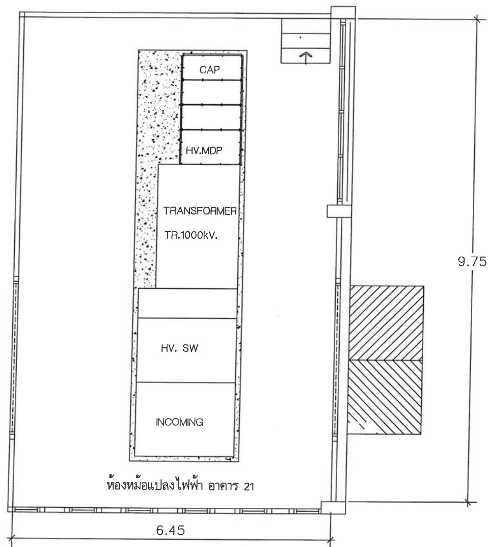
แบบแสดงตำแหน่งตู้ HV. Switch ของเดิมที่จะทำการเปลี่ยน หน่วยเป็น เมตร
