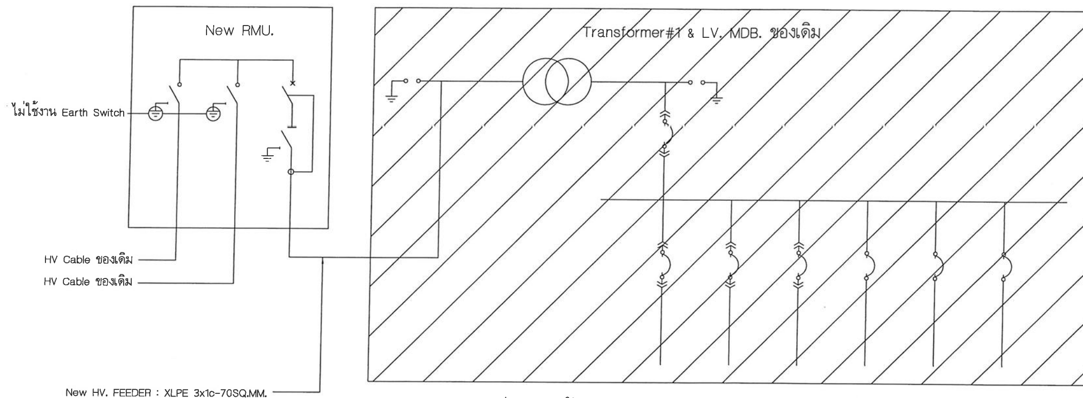
SINGLE LINE DIAGRAM ระบบจ่ายไฟฟ้า อาคาร 21 ภายหลังการปรับปรุง
