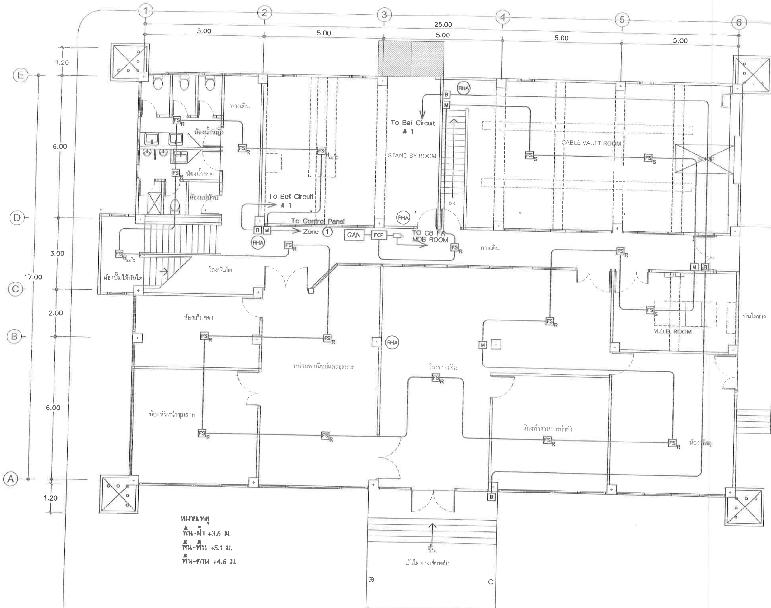
แปลนพื้นที่ 1 อาคารหอพักนักเรียน(อาคารใหม่) มาตรฐาน
