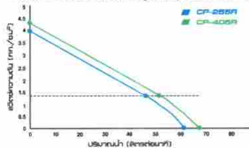
กราฟแสดงสมรรถนะปั้มน้ำอัตโนมัติ WP ในรุ่นธรรมดา (CP)
