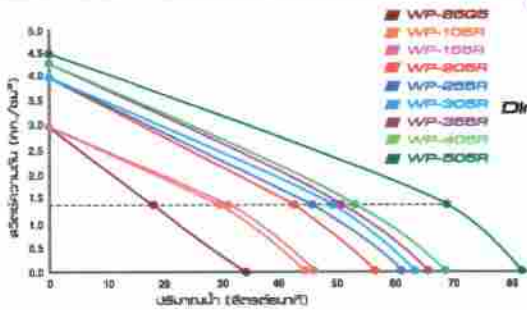
กราฟแสดงสมรรถนะปั้มน้ำอัตโนมัติ WP ในรุ่นอัตโนมัติ (WP)
