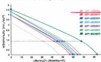
การไหลของน้ำในระบบน้ำอัตโนมัติ (EP)
