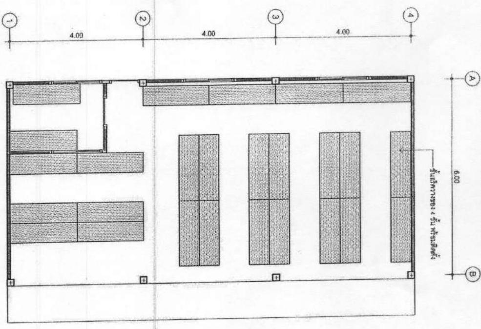
แปลนวางชิ้นวางของ 1:75
