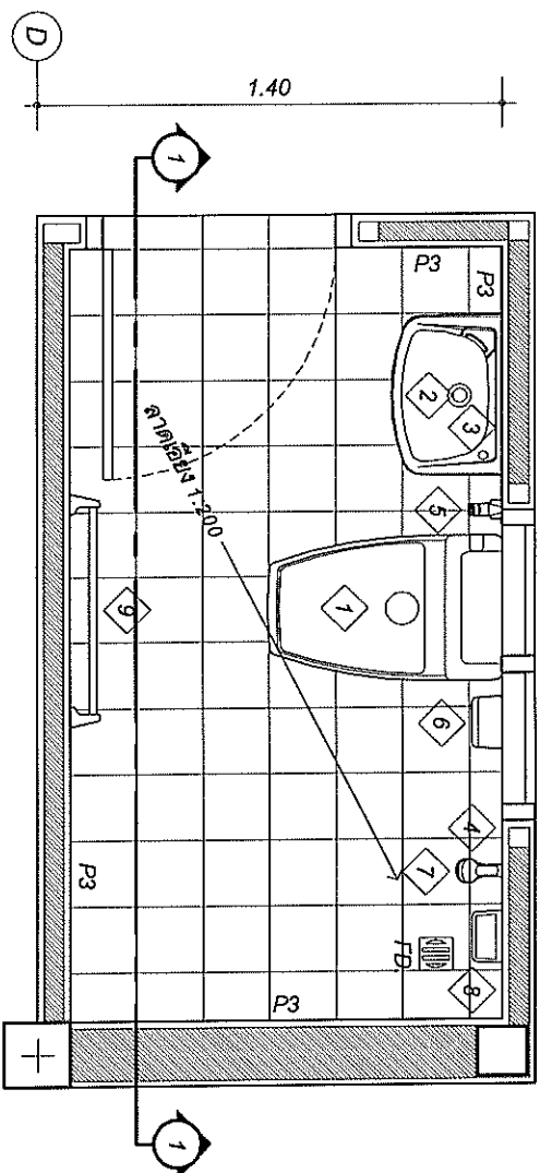
แบบขยายห้องน้ำ 1 1:25
