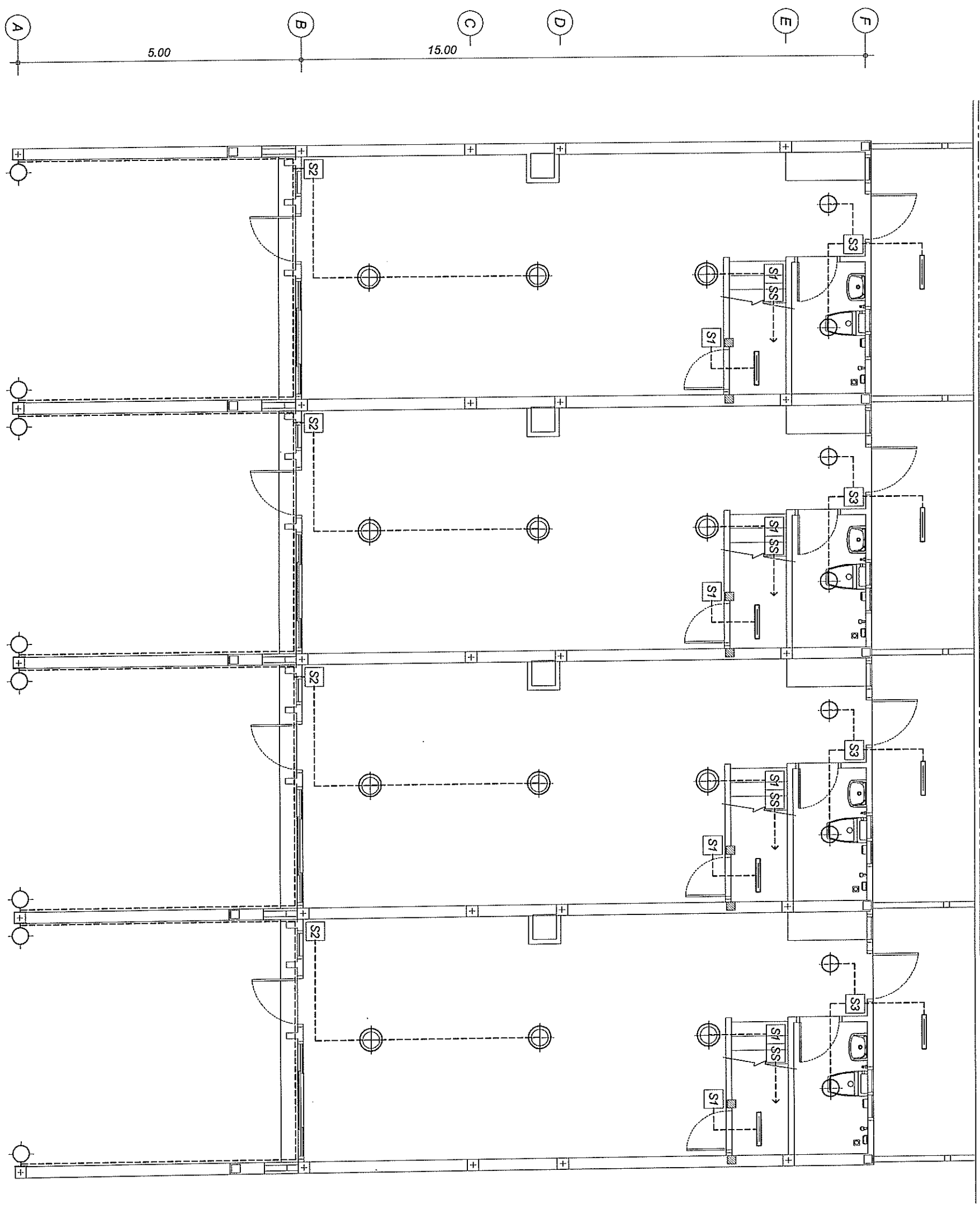
แปลนไฟฟ้าส่องสว่าง ชั้นล่าง 1:75
