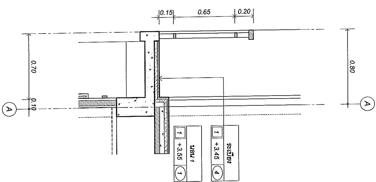
รูปตัด 1-1 1:25
