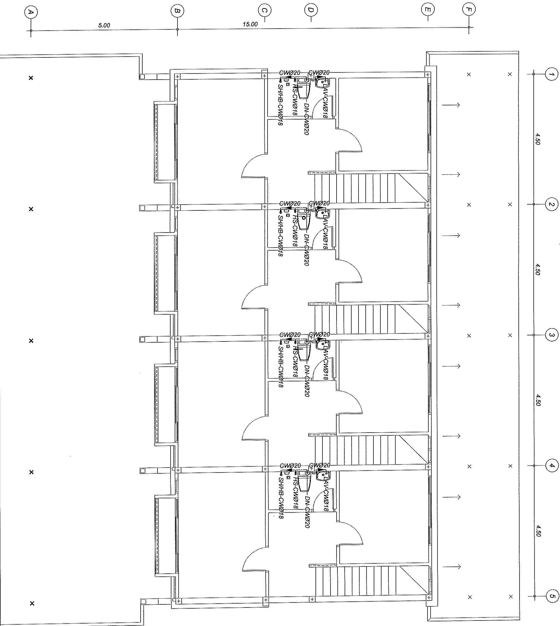
แปลนระบบประปา ชั้น 2 1:75
