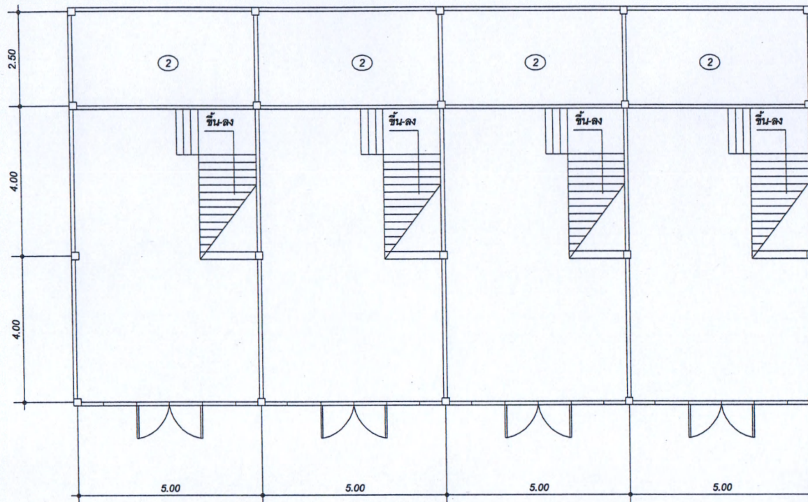
แปลนพื้นที่ชั้นล่าง หลังที่ 3
