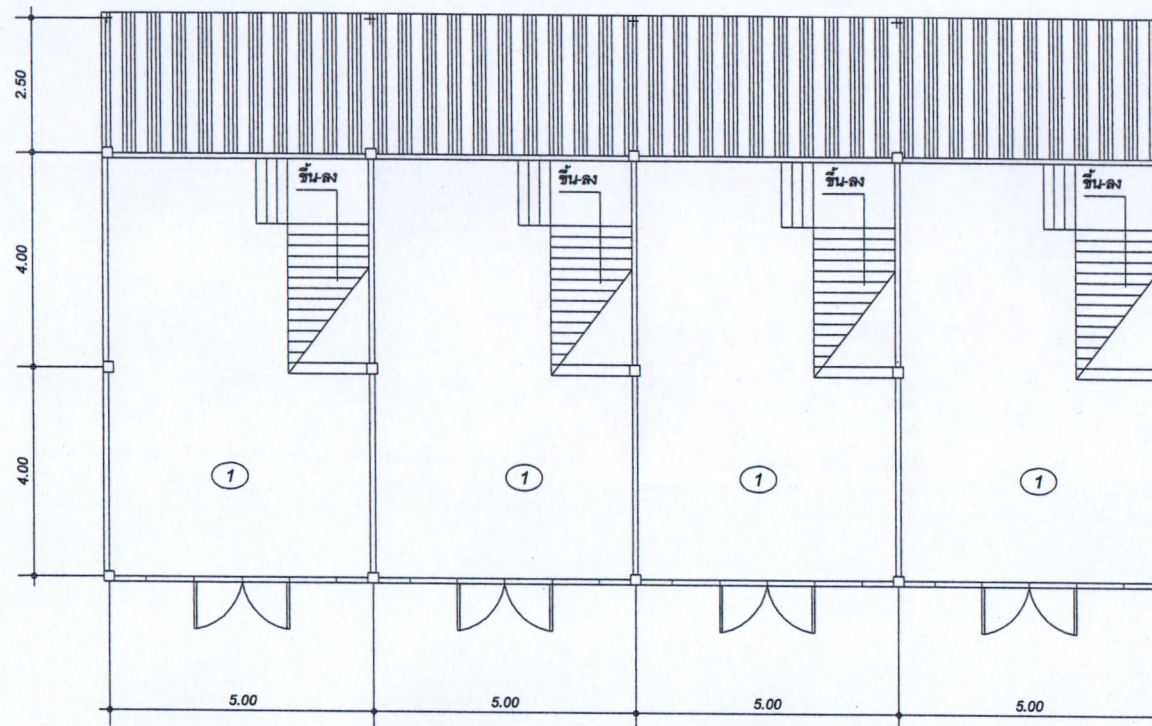
แปลนพื้นที่ชั้นบน หลังที่ 2
