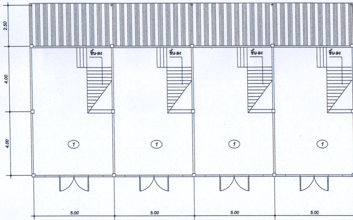
แปลนพื้นที่ชั้นบน หลังที่ 3
