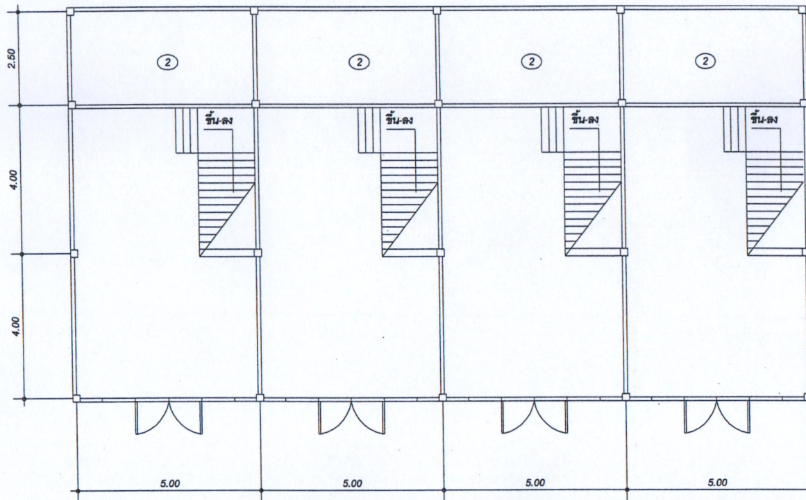
แปลนพื้นที่ชั้นล่าง หลังที่ 2
