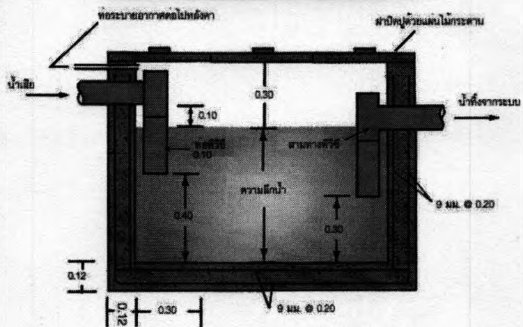
บ่อตกไข่แบบสร้างในที่สำหรับอาคารขนาดใหญ่
