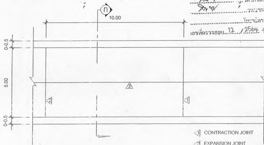
แปลนถนนคอนกรีตเสริมเหล็ก
