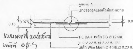
LONGITUDINAL JOINT
