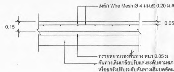
แบบขยายรูปตัดแสดงการเสริมเหล็ก
