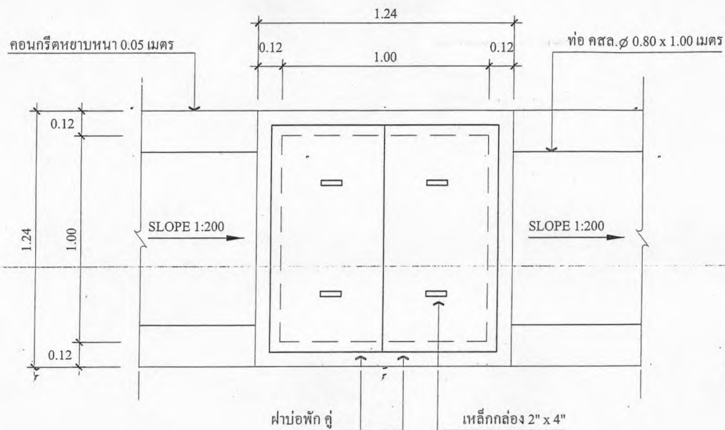
แปลนบ่อพัก NO SCALE
