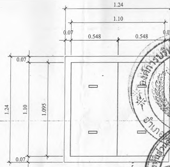
แปลนฝาบ่อพัก NO SCALE
