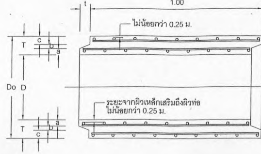
รูปตัดตามยาวแสดงรายละเอียดท่อระบายน้ำ ค.ส.ล. แบบปากลิ้นราง ไม่แสดงมาตราส่วน
