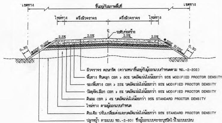
รูปตัดแสดงโครงสร้างถนนคอนกรีตเสริมเหล็กและคูลงบผิววัสดุ
