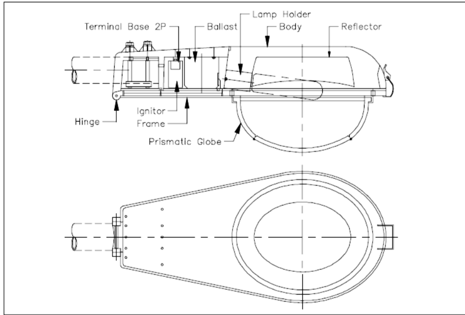
รูปที่ ๑-๑ แสดงโคมไฟฟ้า (Luminaire) ที่ประกอบด้วยหลอดไฟฟ้า และชุดประกอบเพื่อติดตั้งให้แสงสว่างแก่บริเวณที่ต้องการ
