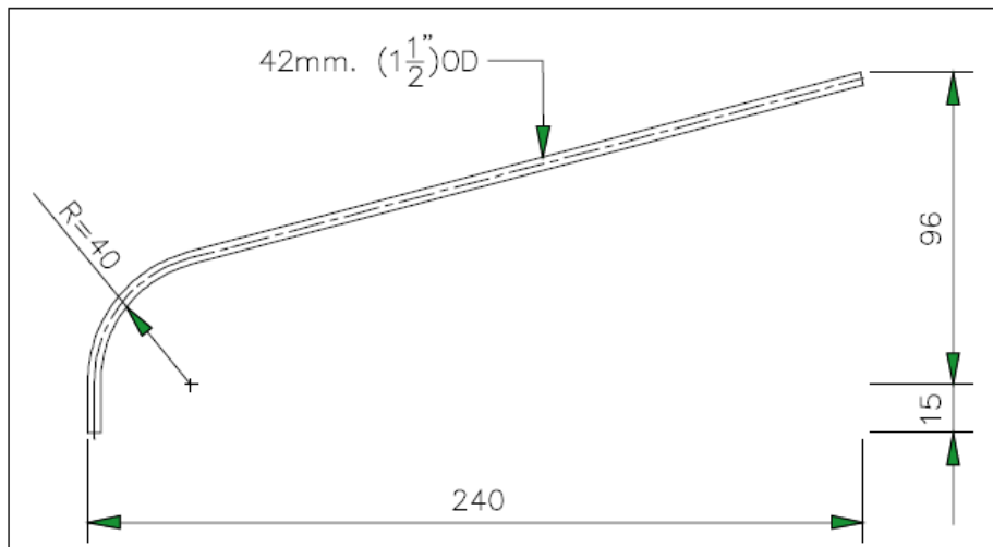
รูปที่ ๑-๓ กิ่งโคมไฟฟ้า (Rod หรือ Arm) อุปกรณ์ที่เชื่อมต่อกับโคมไฟฟ้า และแป้นติดกิ่งโคมเพื่อยื่นออกไปให้แสงสว่างแก่บริเวณที่ต้องการ
