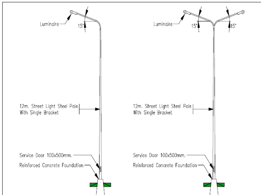
รูปที่ ๑-๒ แสดงชุดโคมไฟถนน
