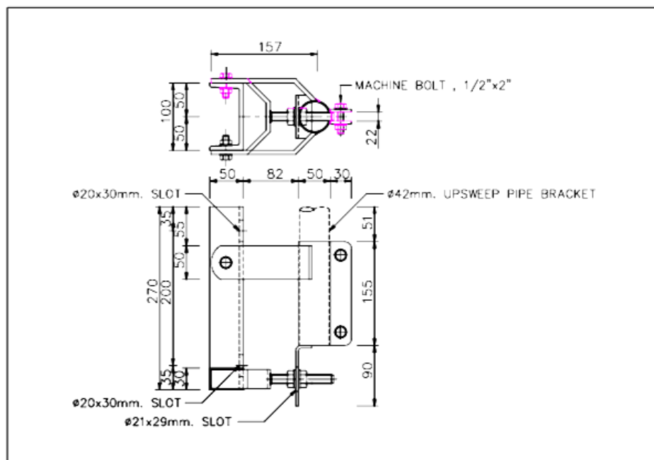
รูปที่ ๑-๔ แป้นติดกิ่งโคม (Bracket) อุปกรณ์ที่ติดกับเสาไฟฟ้า ผนัง หรือกำแพง เพื่อยึดกิ่งโคมไฟฟ้า และโคมไฟฟ้า
