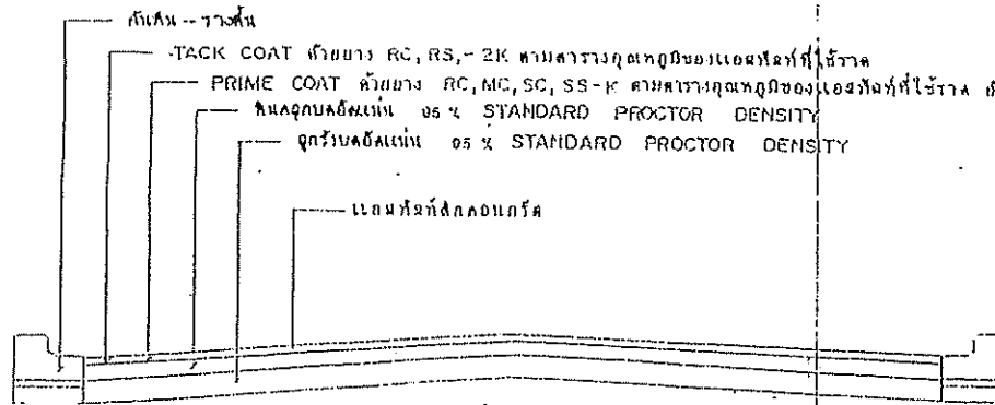
รูปตัดถนน แอสฟัลท์ติก คอนกรีต not to scale
