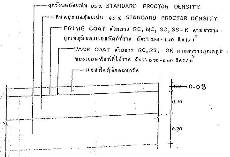
รายละเอียด ASPHALTIC CONCRETE not to scale
