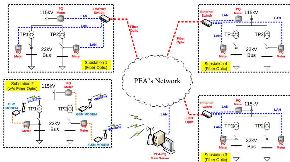
รูปที่ 3.1 ระบบสื่อสารรับ-ส่งข้อมูลระหว่างเครื่องวัดฯ มายัง Server ที่ กฟผ. สำนักงานใหญ่
