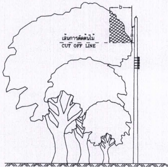
การตัดแต่งต้นไม้สำหรับสายหุ้มฉนวนเต็มพิกัดคิกเลีย TREE TRIMMING FOR TWISTED AERIAL CABLE.
