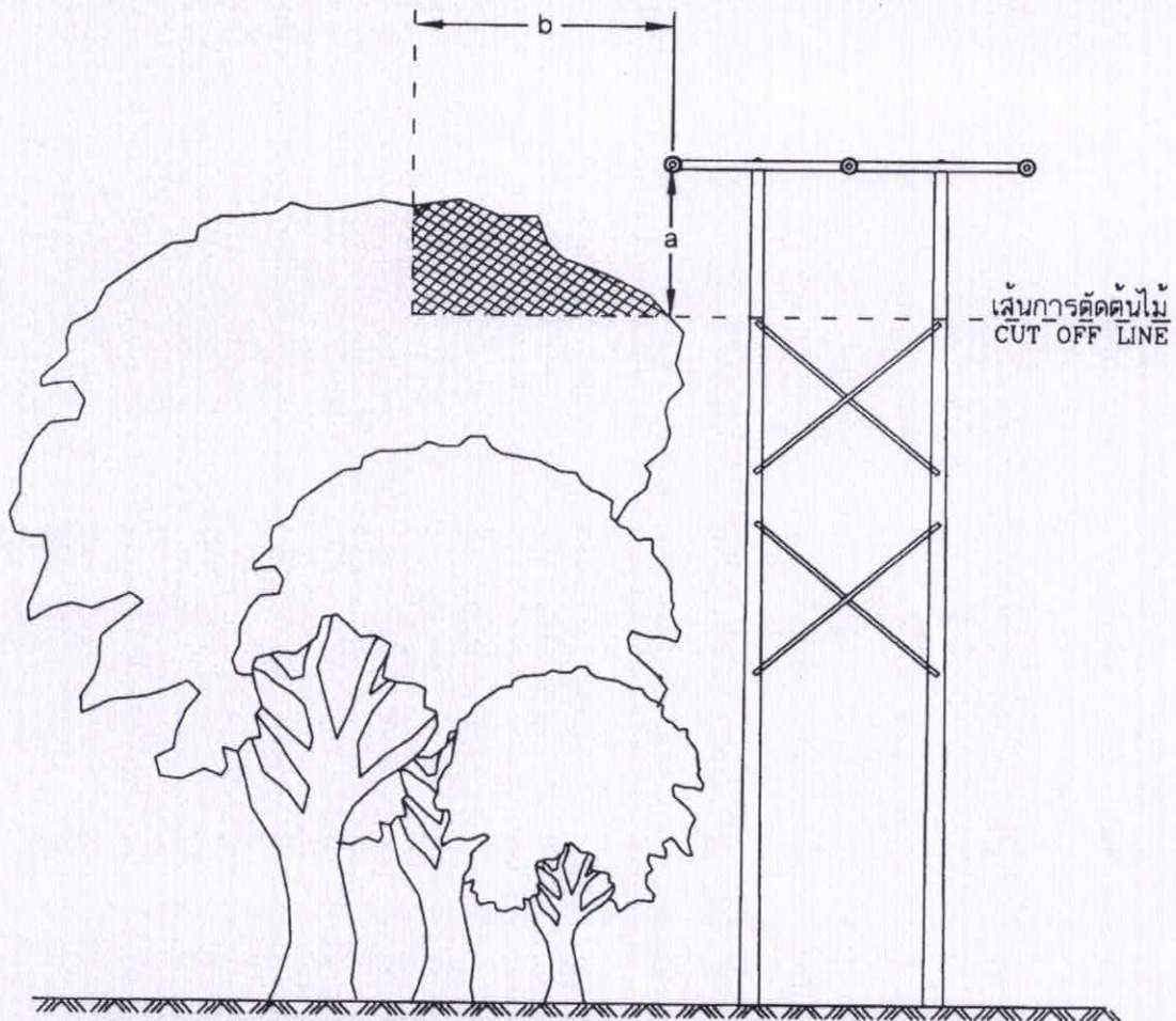
การตัดแต่งต้นไม้สำหรับสายเปลือยแรงสูงที่มีระยะทางระหว่างเสาดั้งแต่ 100 เมตร ขึ้นไป TREE TRIMMING FOR H.V. BARE CONDUCTOR WITH SPANS OF 100 m AND ABOVE.
