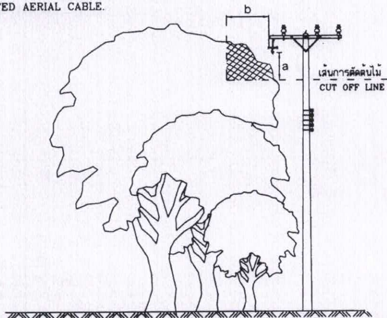
การตัดแต่งต้นไม้สำหรับสายหุ้มฉนวนแบบไม่เต็มพันคดหรือเคเบิลอากาศ TREE TRIMMING FOR PARTIALLY INSULATED CONDUCTOR OR SPACED AERIAL CABLE.
