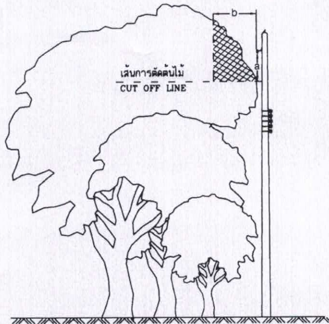
การตัดแต่งต้นไม้สำหรับสายหุ้มฉนวนเดิมพันคดเกลียว TREE TRIMMING FOR TWISTED AERIAL CABLE.
