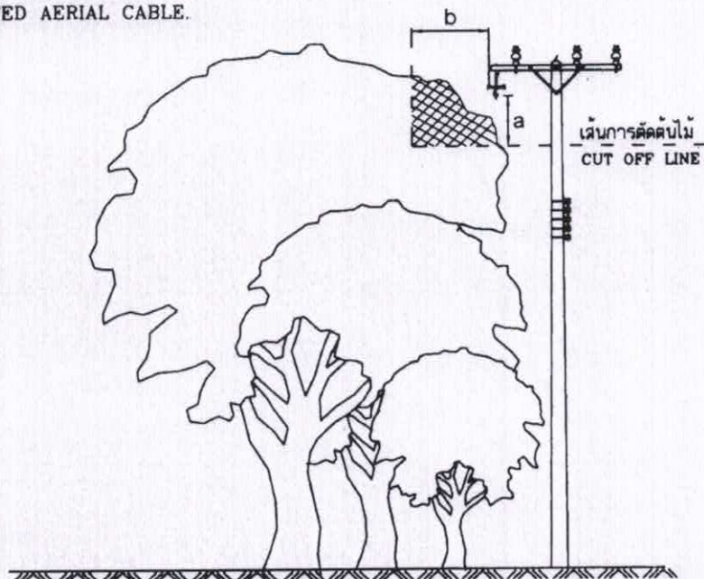
การตัดแต่งต้นไม้สำหรับสายหุ้มฉนวนแบบไม่เดิมพันคดหรือเคเบิลอากาศ TREE TRIMMING FOR PARTIALLY INSULATED CONDUCTOR OR SPACED AERIAL CABLE.
