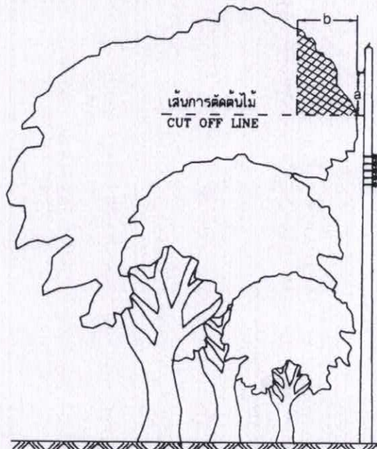
การตัดแต่งต้นไม้สำหรับสายหุ้มฉนวนเต็มพิกัดตีเกลียว TREE TRIMMING FOR TWISTED AERIAL CABLE.
