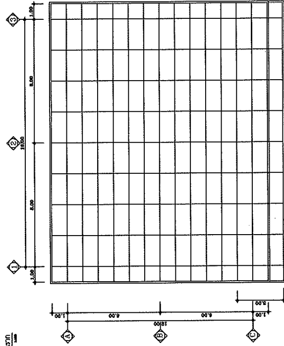
แบบแปลนบริเวณ Floor Plan
