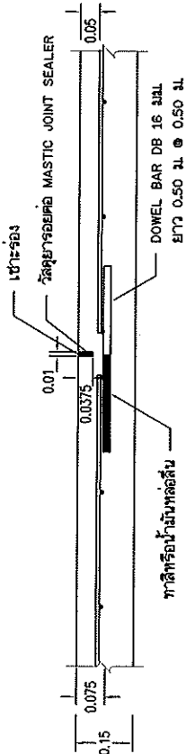
ขยายรอยต่อ CONSTRUCTION JOINT (ทุก 10.00 ม.) NOT TO SCALE
