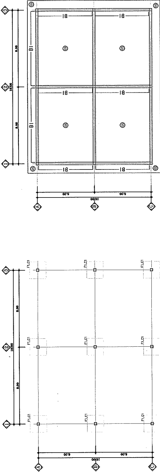
แบบแปลนพื้นที่ Floor Plan
