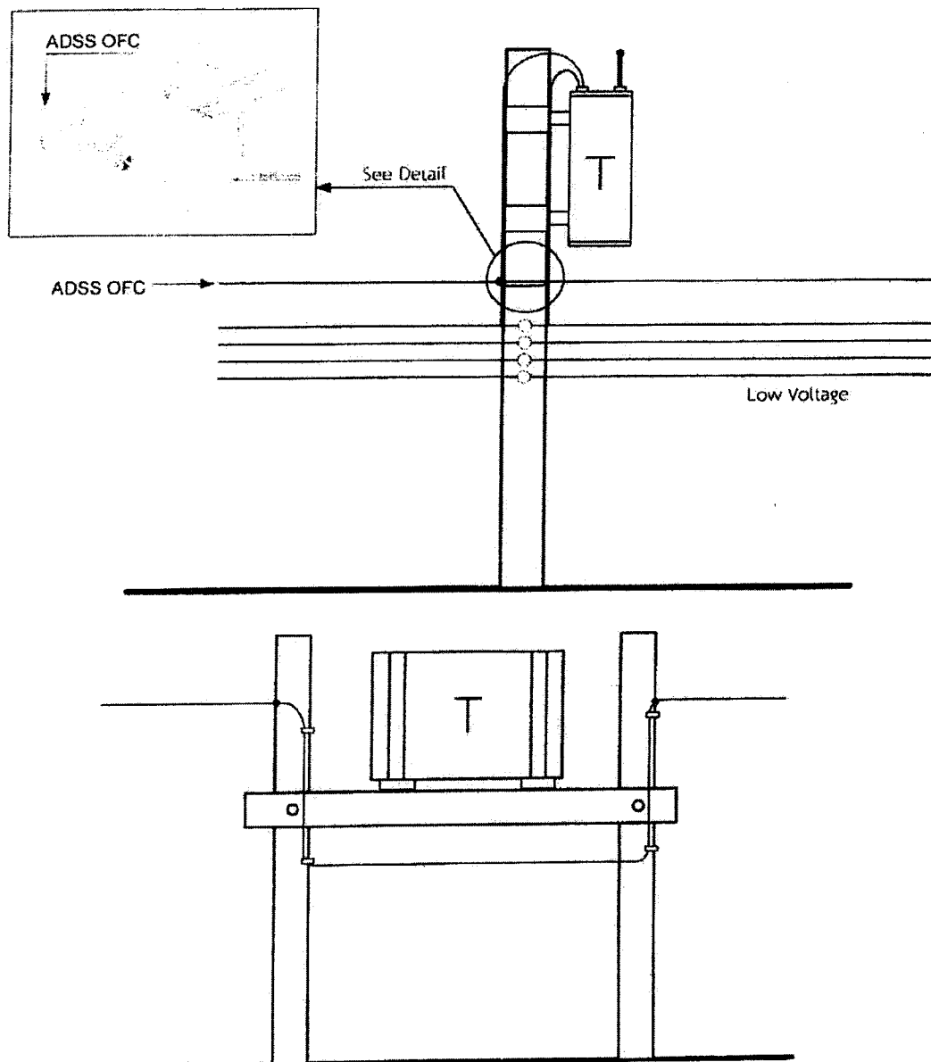
รูปที่ 2 แสดงการติดตั้ง Extension Arm ที่เสาหม้อแปลงเดี่ยวและหม้อแปลงคู่
