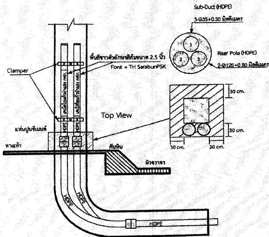
รูปที่ 10.1 การระบุชื่อ กฟภ. บนท่อ Riser
