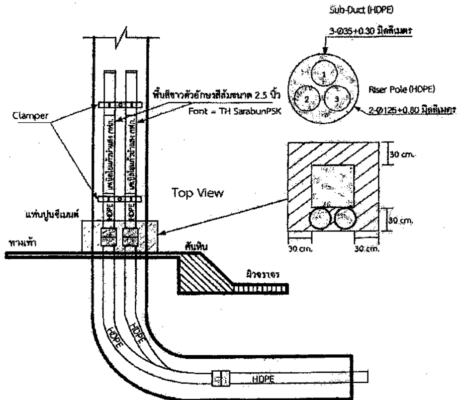
รูปที่ 10.1 การระบุชื่อ กฟผ. บนท่อ Riser
