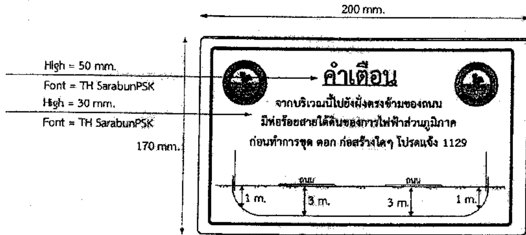
รูปที่ 10.2 ป้ายระบุตำแหน่งท่อร้อยสายเคเบิลใยแก้วนำแสง
