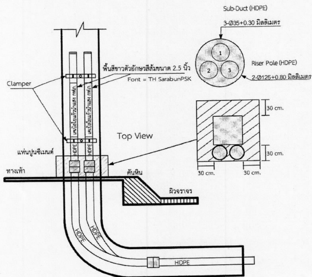
รูปที่ 10.1 การระบุชื่อ กฟภ. บนท่อ Riser
