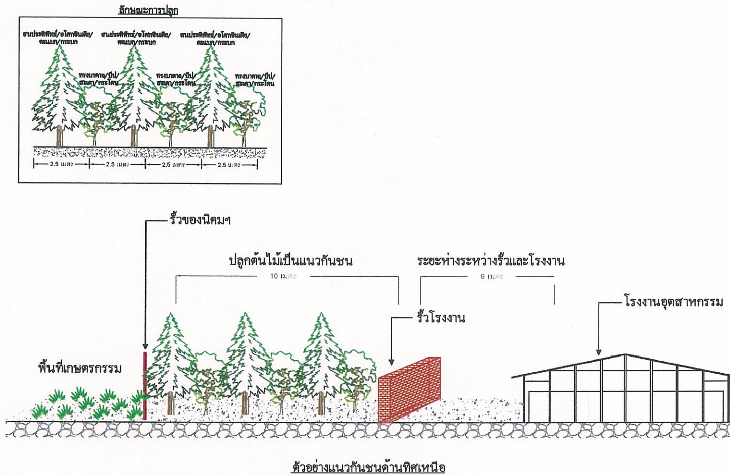
รูปที่ 2-1 (ต่อ) ผังแม่บทและพื้นที่สีเขียวของโครงการ
