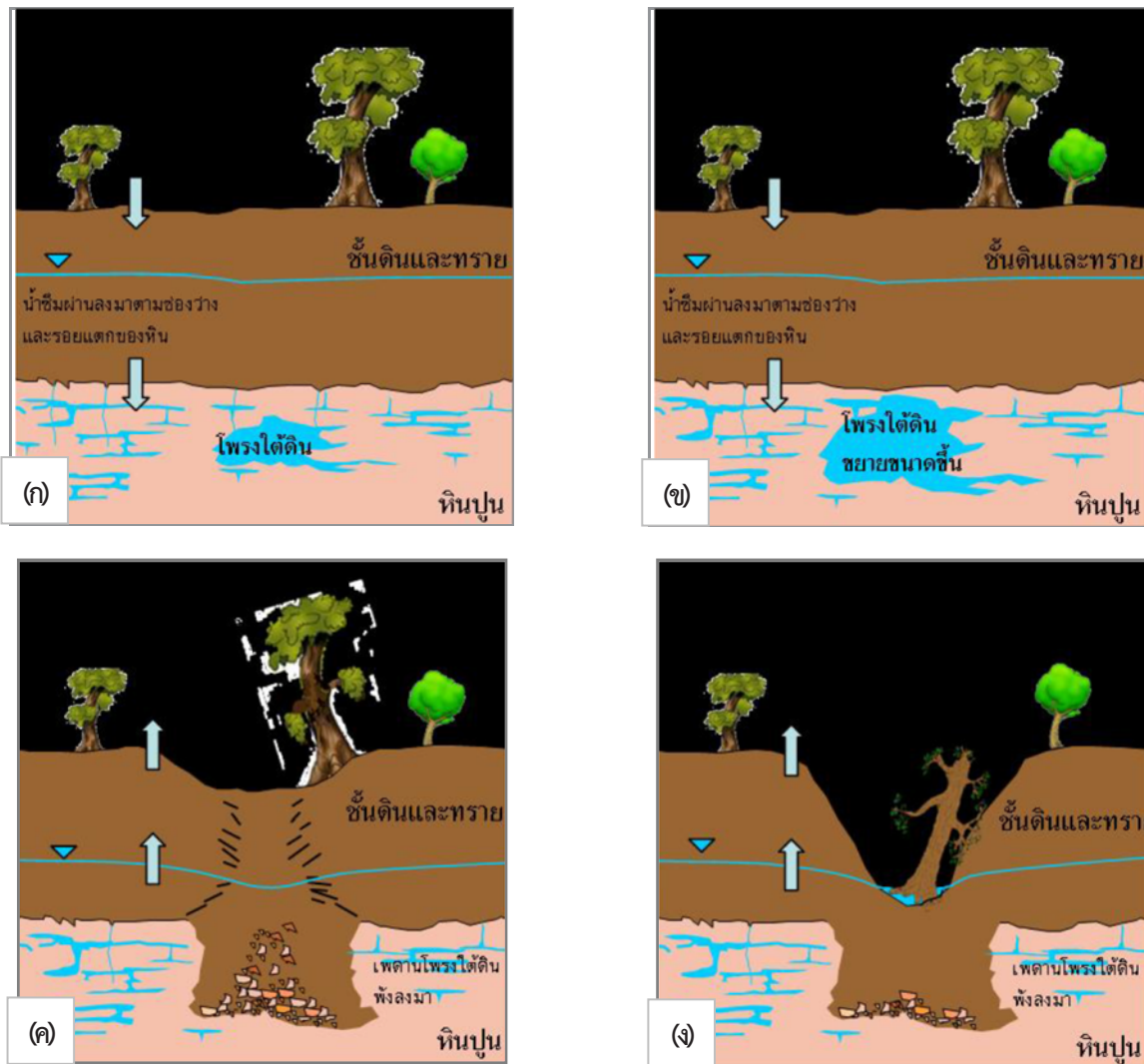
รูปที่ 4-4 แบบจำลองการเกิดหลุมยุบ (กรมทรัพยากรธรณี www.dmr.go.th คัดลอกจาก ศิริประภา ชาติประเสริฐ, 2551)
