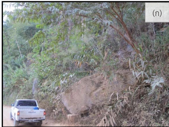
รูปที่ 3-7 ลักษณะของหินยุคดีโวเนียน
