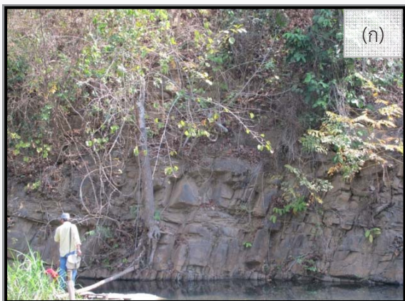
รูปที่ 5-15 ลักษณะกลุ่มหินห้วยโป่ง ยุคไทรแอสซิก ตำบลห้วยโป่ง อำเภอเมืองแม่ฮ่องสอน
