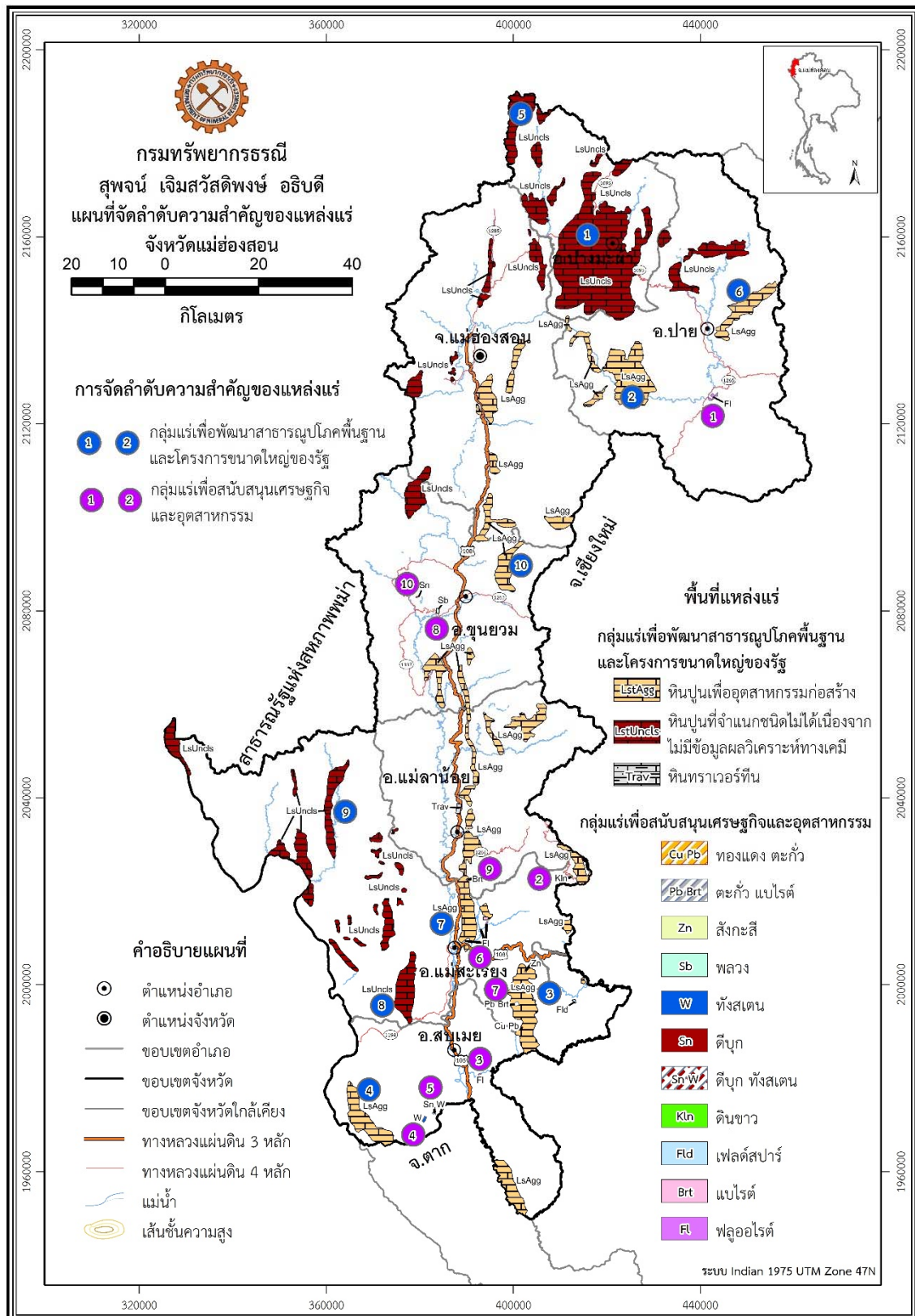
รูปที่ 6-15 แผนที่แสดงลำดับความสำคัญของแหล่งแร่ที่พบในจังหวัดแม่ฮ่องสอน ตามกลุ่มแร่การใช้ประโยชน์
