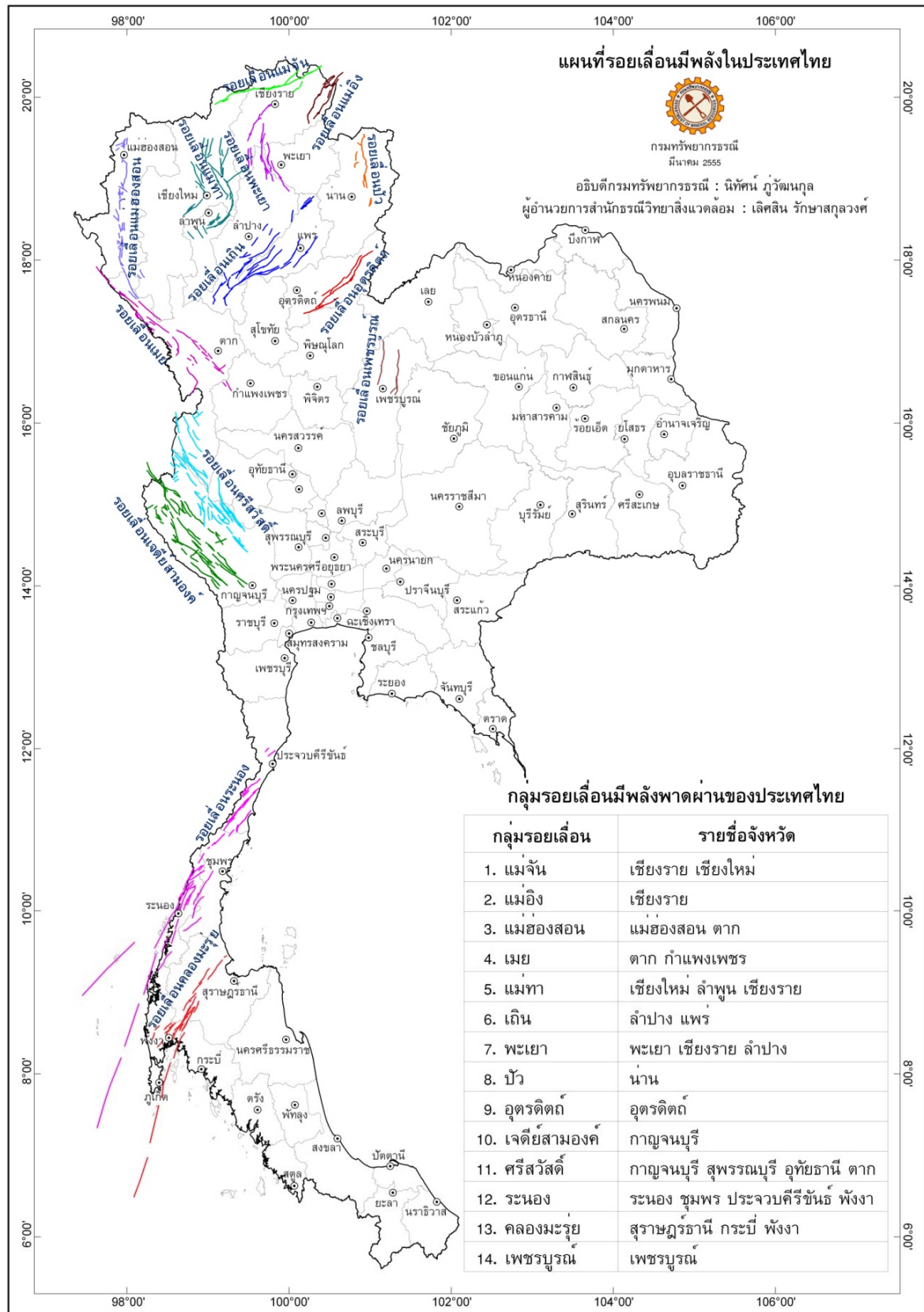
รูปที่ 4-7 แผนที่แสดงแนวรอยเลื่อนมีพลังในประเทศไทย (กรมทรัพยากรธรณี, 2555)
