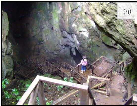
รูปที่ 5-4 ถ้ำผามอน บ้านผามอน ตำบลถ้ำลอด อำเภอปางมะผ้า
