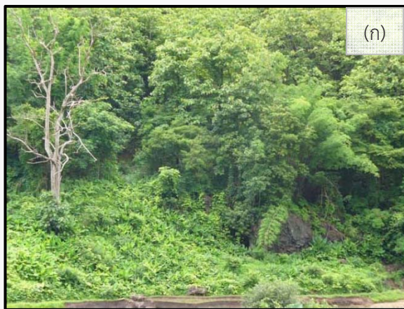
รูปที่ 6-11 ลักษณะแหล่งแร่ฟลูออไรต์น้ำแม่สะเรียง ตำบลป่าแป๋ อำเภอแม่สะเรียง จังหวัดแม่ฮ่องสอน
