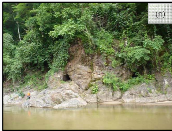
รูปที่ 6-4 ลักษณะแหล่งแร่ทองแดงและตะกั่วบ้านห้วยวอก ตำบลกองก้อย อำเภอสะเมิง จังหวัดแม่ฮ่องสอน
