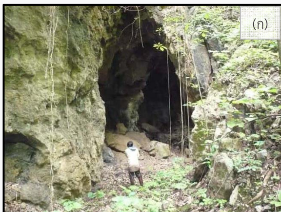
รูปที่ 6-14 ลักษณะแหล่งแร่ฟลูออไรต์น้ำแมริด ตำบลแม่สวด อำเภอสบเมย จังหวัดแม่ฮ่องสอน
