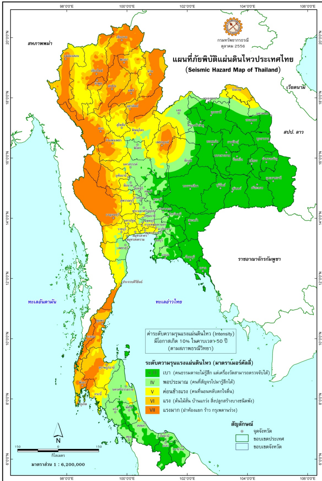
รูปที่ 4-8 แผนที่ภัยพิบัติแผ่นดินไหวประเทศไทย (กรมทรัพยากรธรณี, 2556ก)
