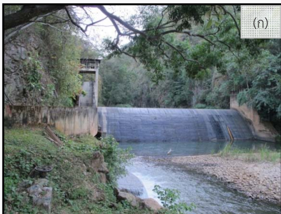
รูปที่ 3-2 หมวดหินผาบ่อง ยุคแคมเบรียน บริเวณเขื่อนผาบ่อง ตำบลผาบ่อง อำเภอเมืองแม่ฮ่องสอน
