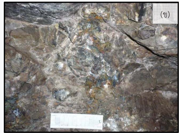
รูปที่ 6-4 ลักษณะแหล่งแร่ทองแดงและตะกั่วบ้านห้วยวอก ตำบลกองก้อย อำเภอสะเมิง จังหวัดแม่ฮ่องสอน
