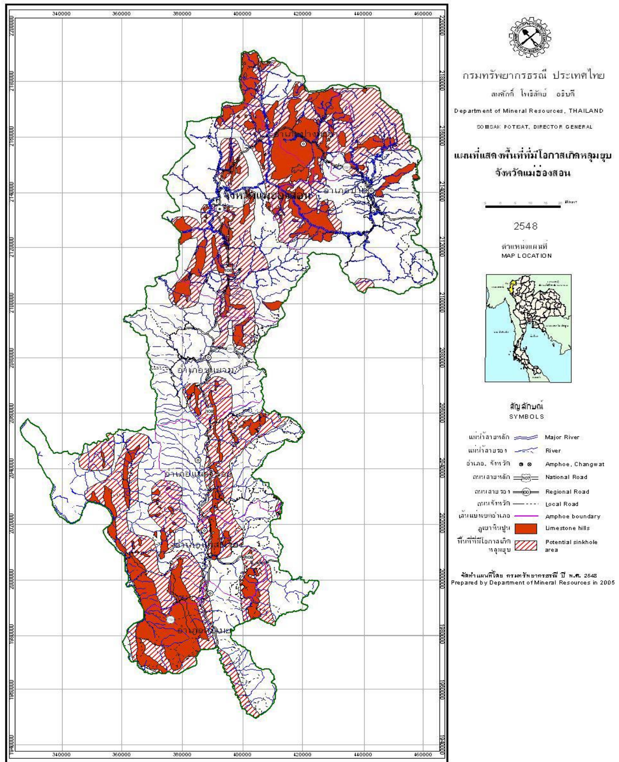
รูปที่ 4-5 แผนที่แสดงพื้นที่ที่มีโอกาสเกิดหลุมยุบ จังหวัดแม่ฮ่องสอน (กรมทรัพยากรธรณี, 2548)
