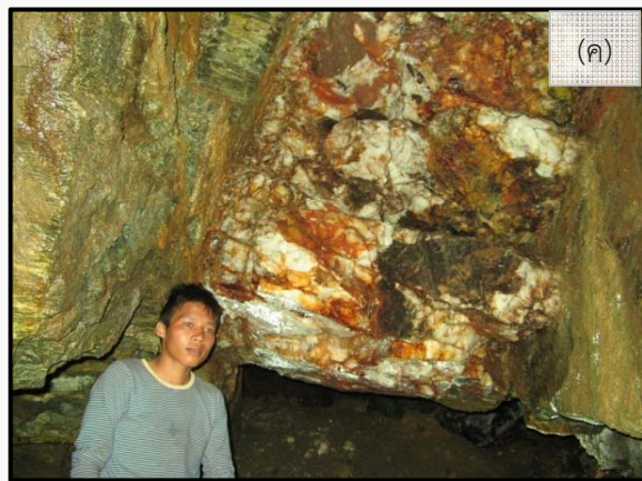
รูปที่ 6-6 ลักษณะแหล่งแร่ทั้งสแตนเหมืองแม่ลาม่า ตำบลสบเมย อำเภอสบเมย จังหวัดแม่ฮ่องสอน
