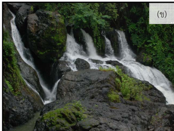
รูปที่ 5-7 น้ำตกผาเสือ เขตอุทยานแห่งชาติถ้ำปลา-น้ำตกผาเสือ ตำบลหมอกจำแป่ อำเภอเมืองแม่ฮ่องสอน
