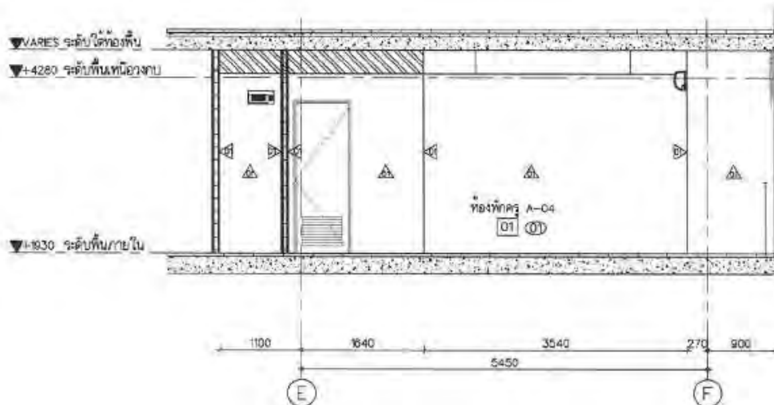
รูปด้าน 01:RENOVATION PLAN:แบบขยาย ห้องพัสดุ A-04 มาตราส่วน 1:50
