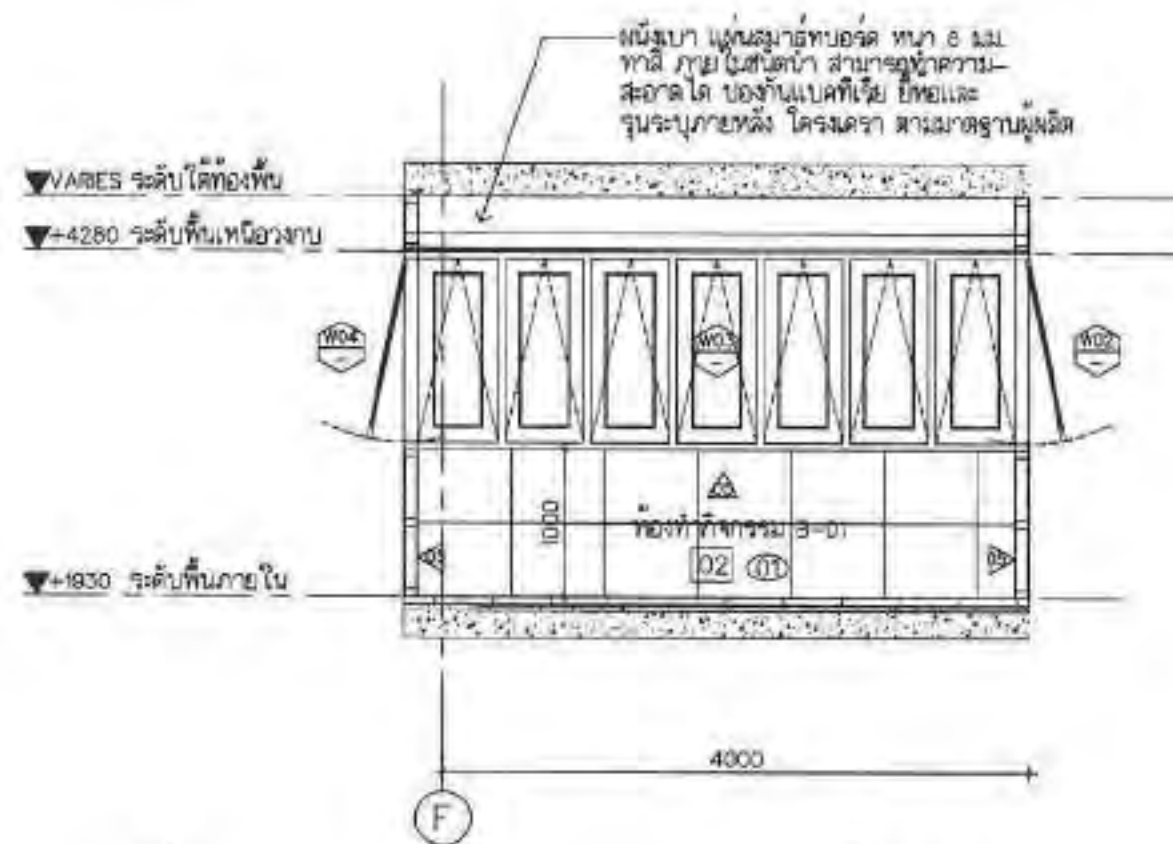
รูปด้าน 04 RENOVATION PLAN:แบบขยาย ห้องทำกิจกรรม B-01 หน้า 130
