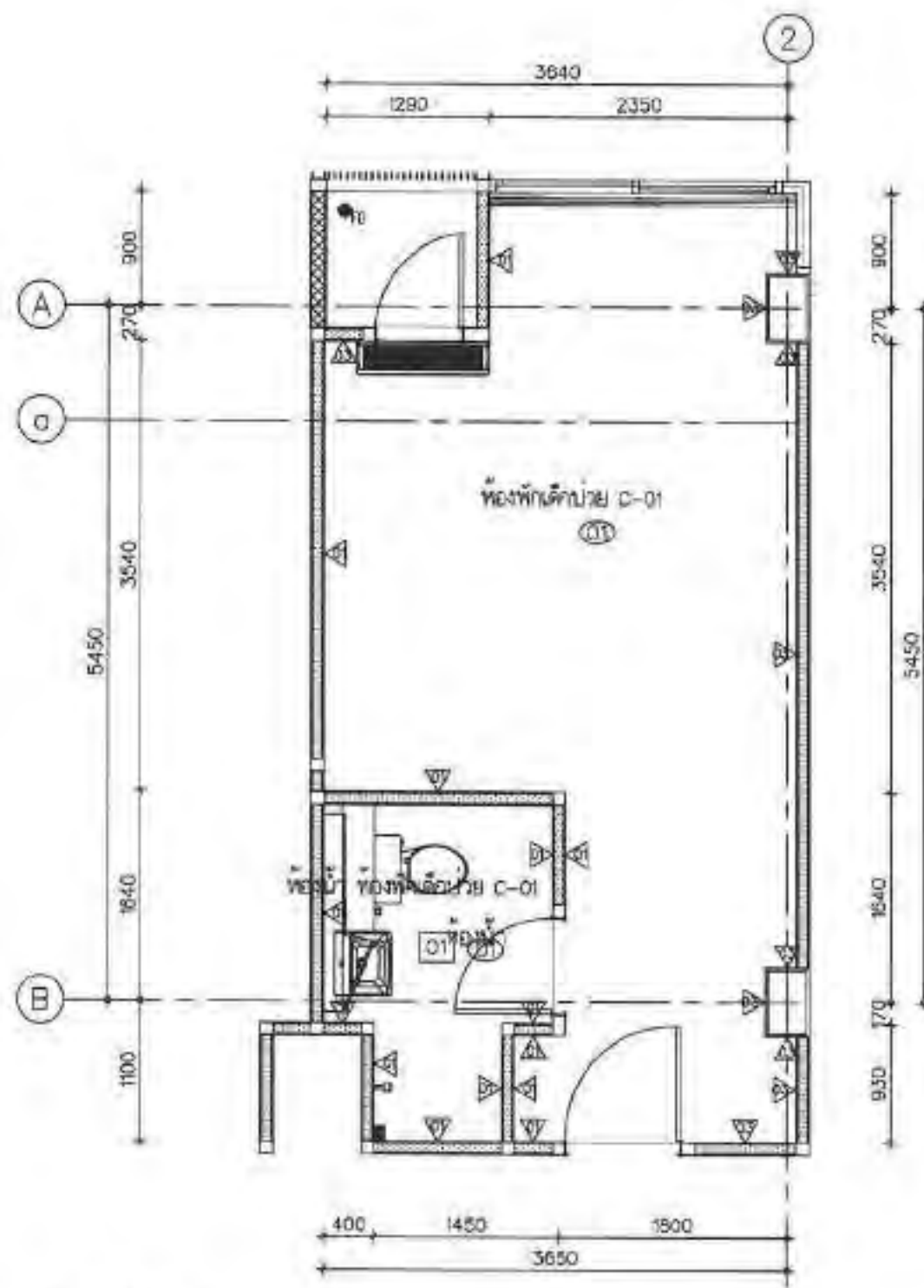
RENOVATION PLAN: แบบขยาย ห้องพักเด็กป่วย C-01 1/100
