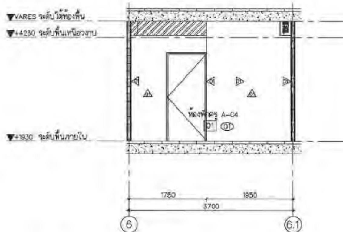
รูปด้าน 01:RENOVATION PLAN:แบบขยาย ห้องพัสดุ A-04 มาตราส่วน 1:50
