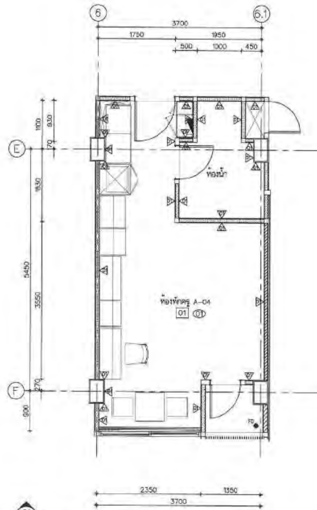
RENOVATION PLAN:แบบขยาย ห้องพัสดุ A-04 มาตราส่วน 1:50
