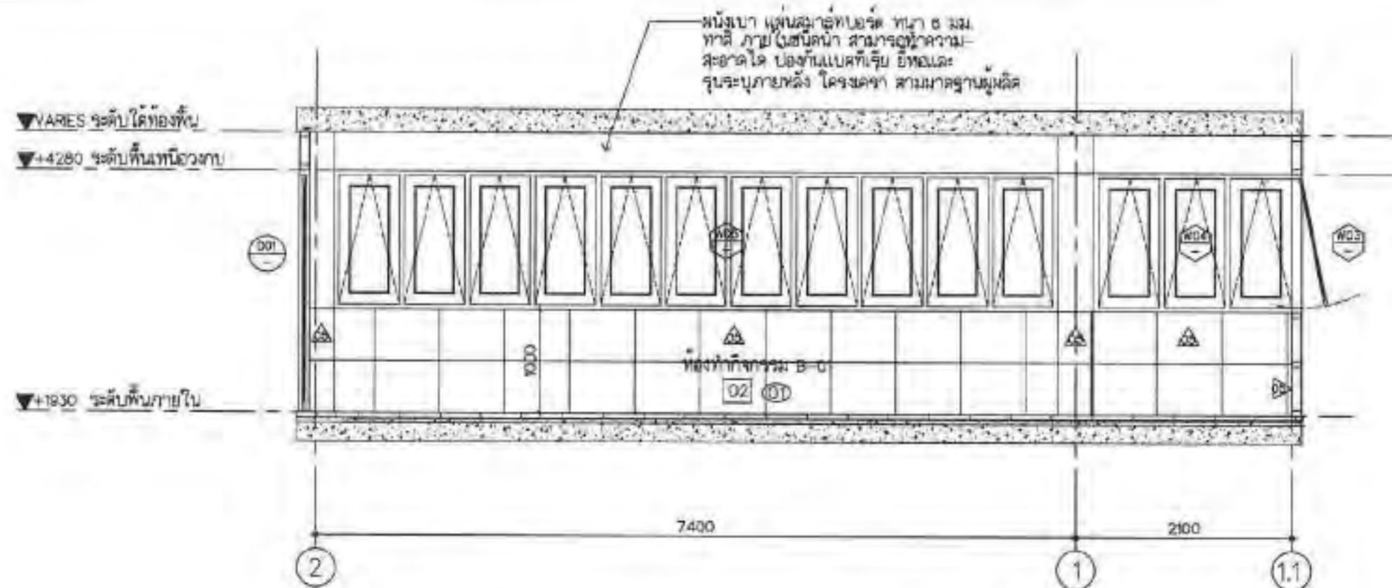
รูปด้าน 03 RENOVATION PLAN:แบบขยาย ห้องทำกิจกรรม B-01 หน้า 130
