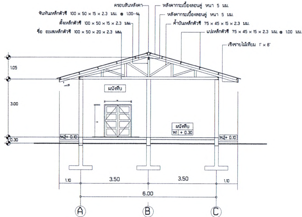
รูปตัด A : A SCALE 1 : 100
