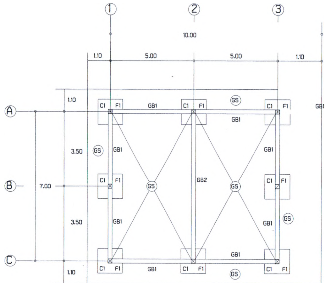
แปลนโครงสร้าง SCALE 1 : 100
