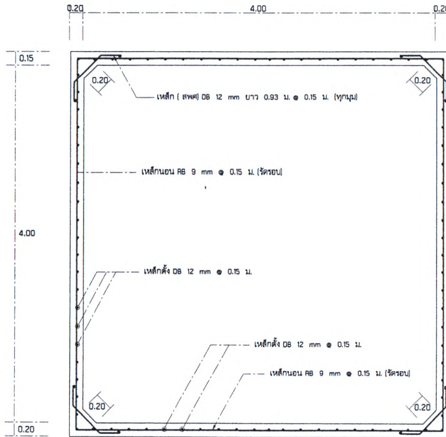
ขยายการเสริมเหล็กผนัง
