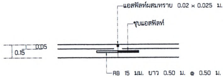
ขยาย CONTRACTION JOINT
