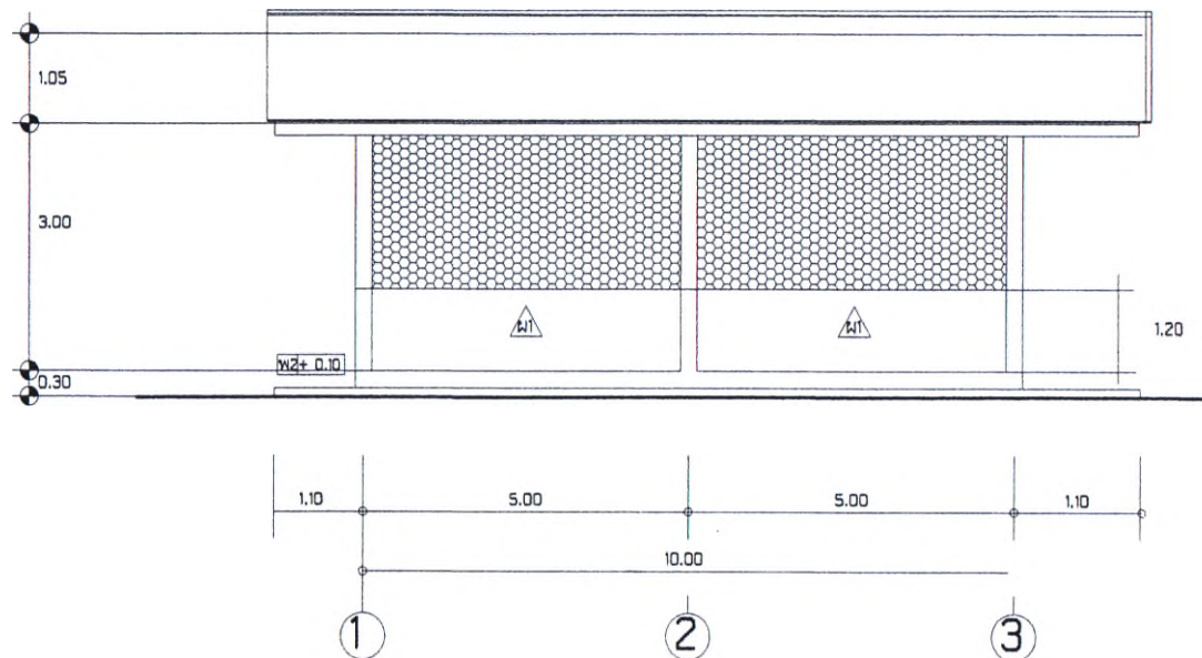
รูปตัด B : B SCALE 1 : 100
