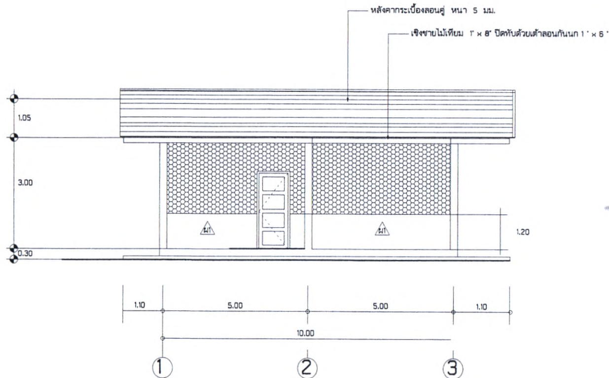
รูปด้าน 1 SCALE 1 : 100
