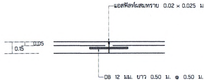
ขยาย LONGITUDINAL JOINT
