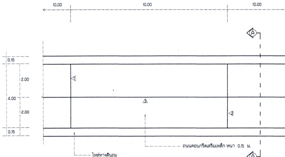
เปลี่ยนถนนคอนกรีตเสริมเหล็ก
