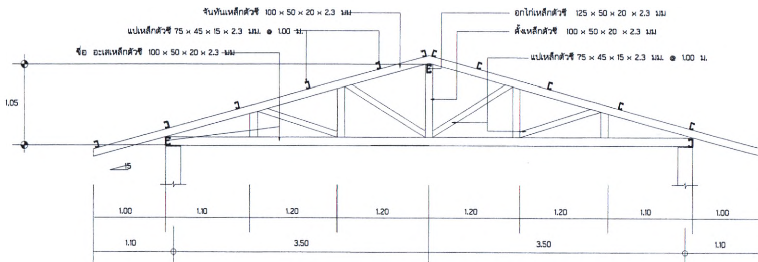
ขยายโครงหลังคา
