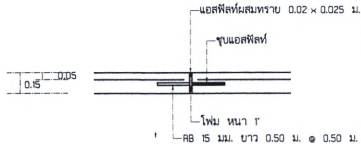
ขยาย EXPANTION JOINT
