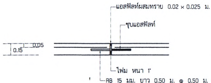
ขยาย EXPANSION JOINT
