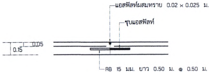
ขยาย CONTRACTION JOINT
