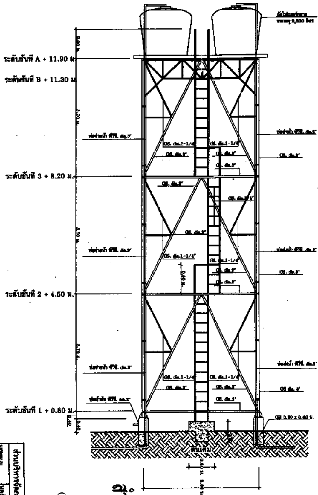
รูปตัดขยายห้องลิฟต์ ขนาด 1:20
