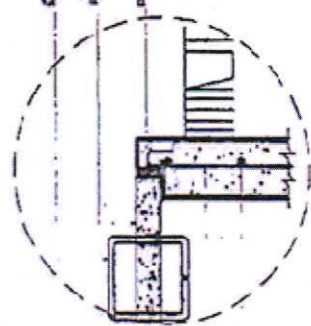
รูปตัด ๑๐-๑๐
