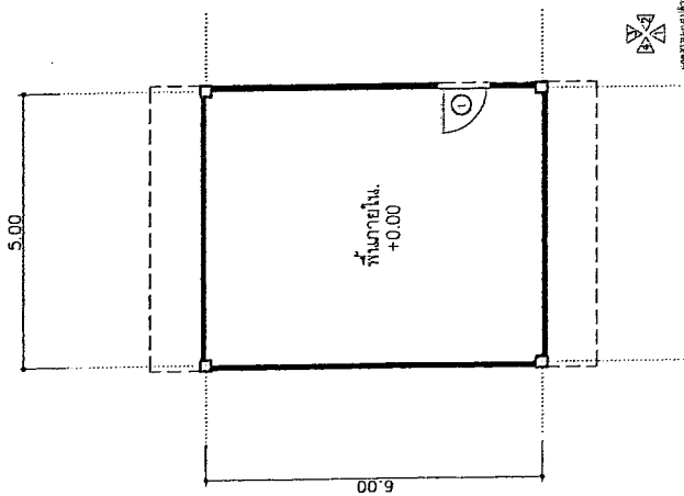
แปลน.
