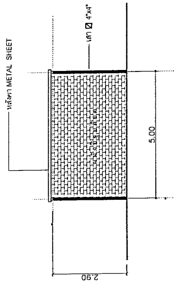
รูปด้านหน้า 1.
