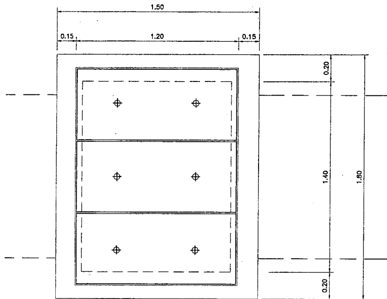
แบบฝาบอพัก
