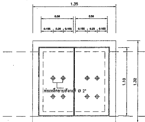
แบบฝาบ่อพัก SCALE 1 : 20
