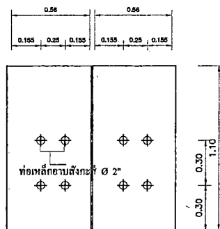
แบบฝาบ่อพัก SCALE 1 : 20
