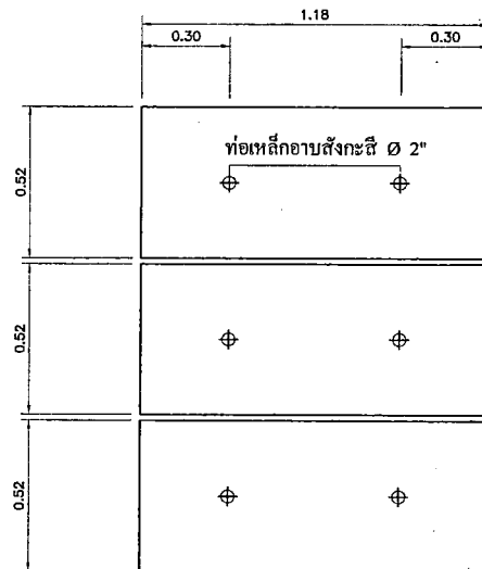
แบบฝาบอพัก
