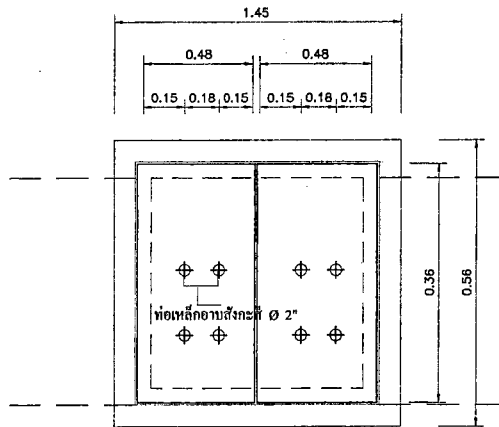
แบบฝาบอพัก
