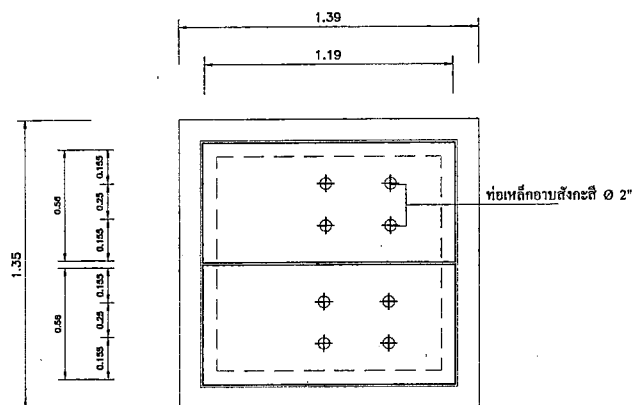
แบบฝาบ่อพัก SCALE 1 : 20
