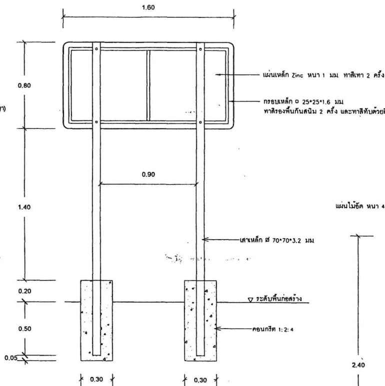
แปลนด้านหลัง ป้ายโครงการ
