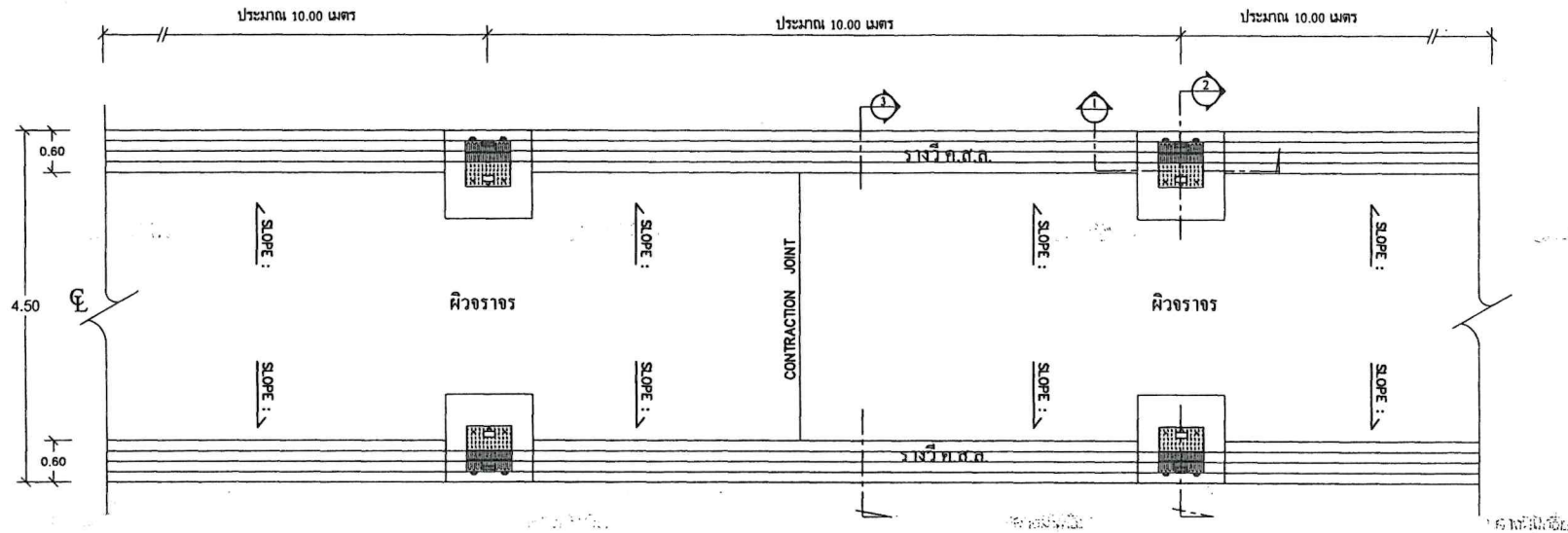
แปลนฝายจราจร กรณีฝายจราจรกว้างน้อยกว่า 5.00 เมตร
