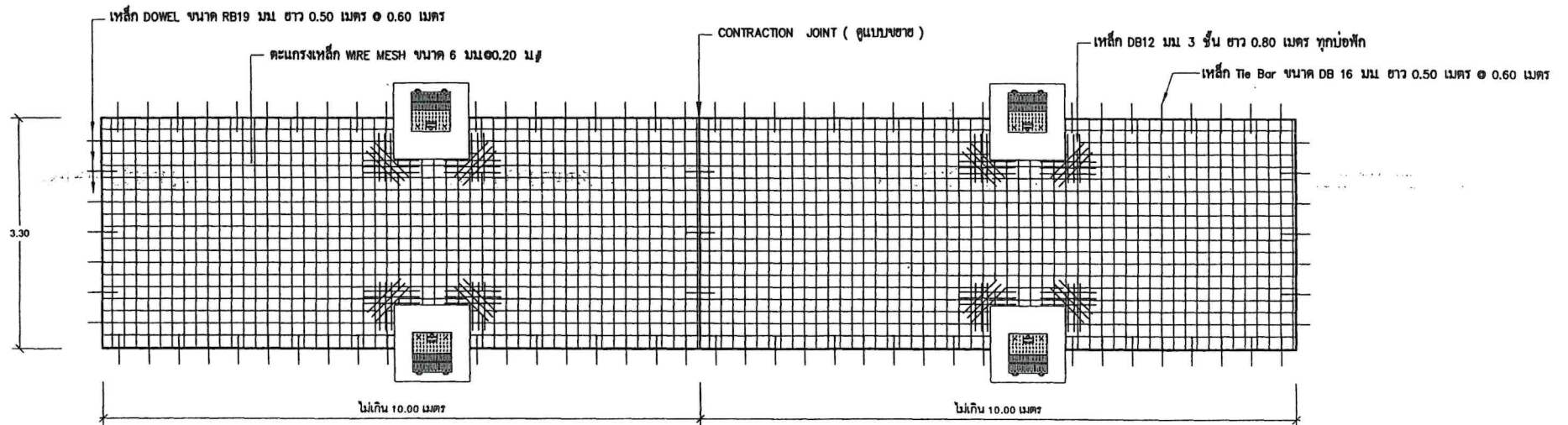
แปลนเสริมเหล็กตะแกรง กรณีฝายจราจรกว้างน้อยกว่า 5.00 เมตร
