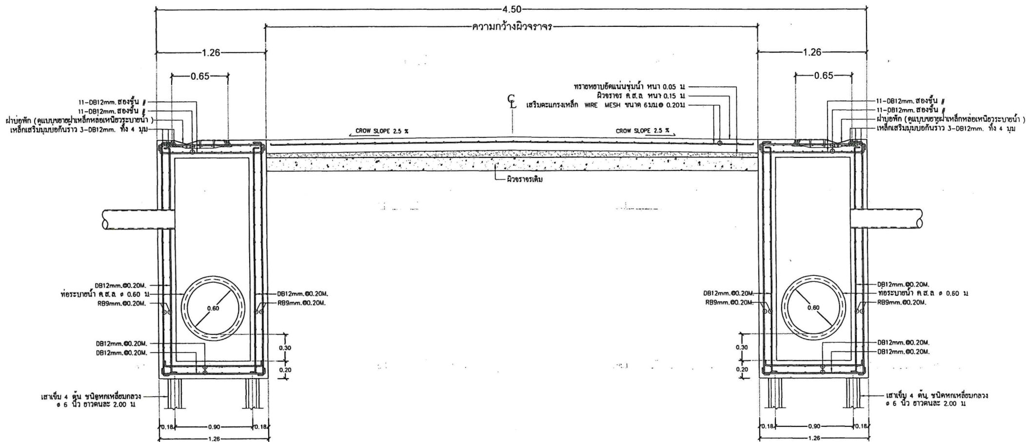
รูปตัด ② สำหรับผิวจราจรกว้างน้อยกว่า 5.00 เมตร มาตราส่วน 1 : 30
