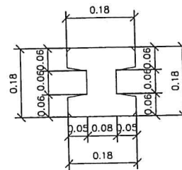
รูปตัดขยายเสาเข็มประตูละบายน้ำ
