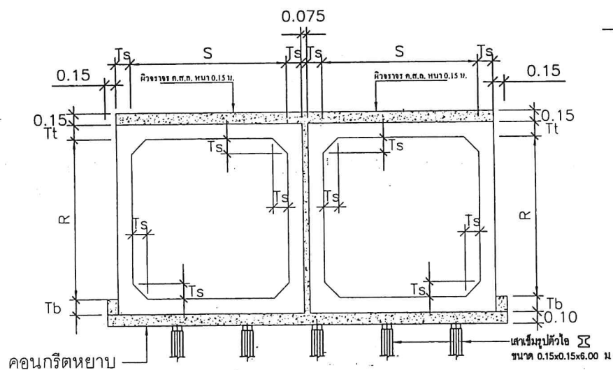
รูปด้าน (ชนิดหลายช่อง) มาตราส่วน 1:50
