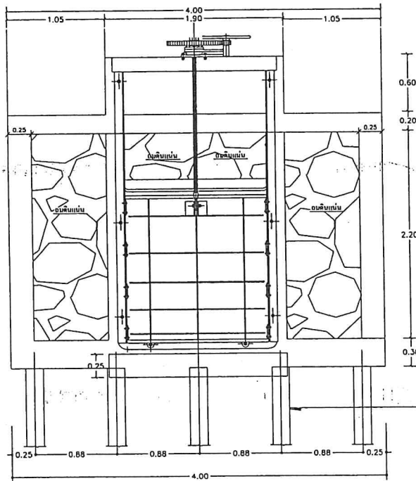
รูปด้านหน้าประตูประบายน้ำ มาตราส่วน 1:40
