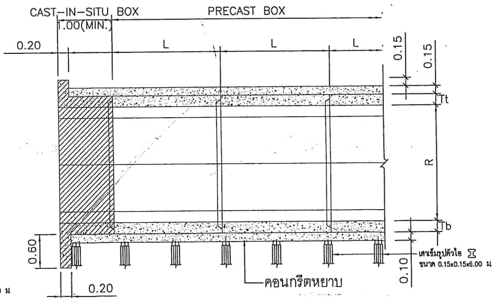
รูปตัดตามยาวของกำแพงปากท่อ มาตราส่วน 1:50
