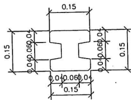
รูปตัดขยายเสาเข็มรางระบายน้ำรูปตัวยู
