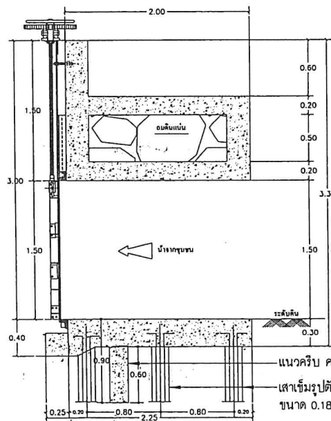
รูปตัดประตูประบายน้ำ มาตราส่วน 1:40
