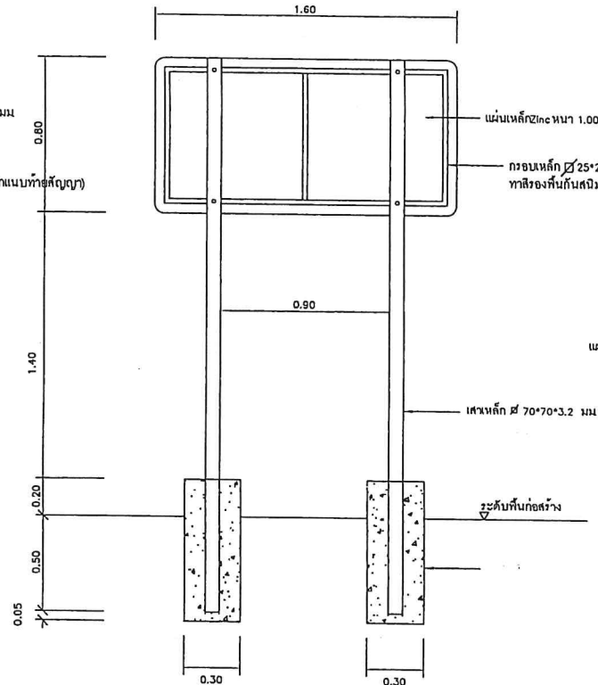
แปลนด้านหลัง ป้ายโครงการ มาตราส่วน 1 : 25
