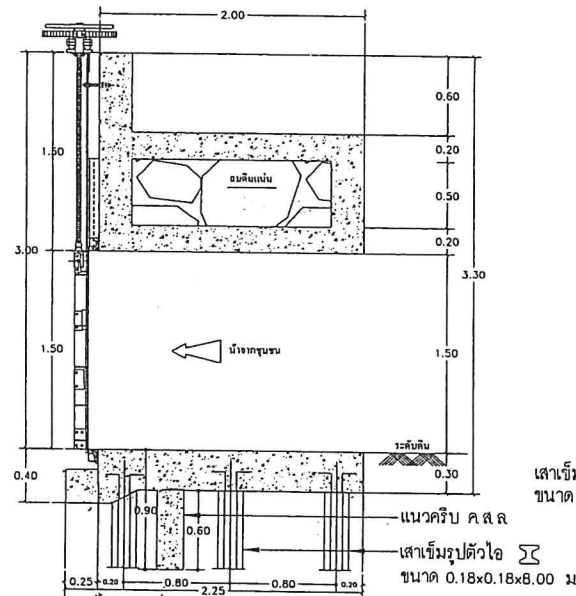
รูปตัดประตูระบายน้ำ มาตราส่วน 1:40
