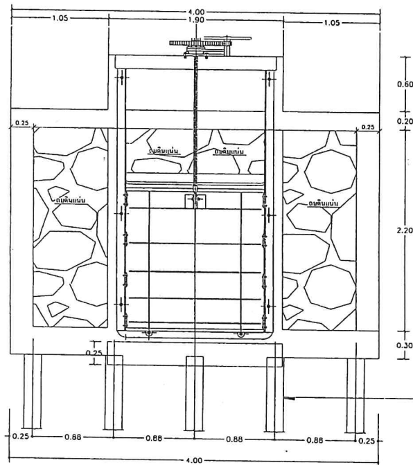
รูปด้านหน้าประตูระบายน้ำ มาตราส่วน 1:40
