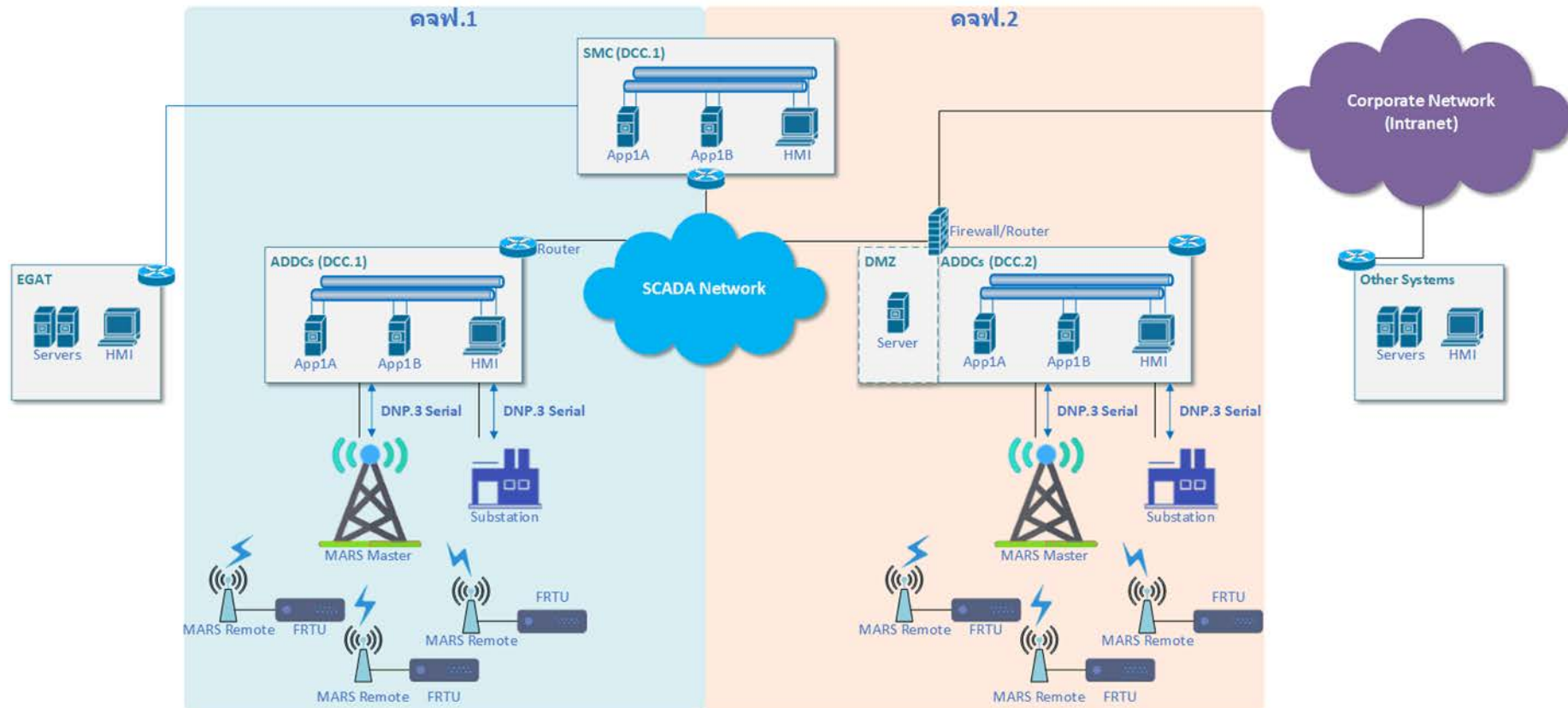
รูปที่ 48 : ภาพแสดงโครงสร้างระบบ SCADA/DMS ตามขอบเขตการควบคุมจ่ายไฟ (คจฟ.) 1 และการควบคุมจ่ายไฟ คจฟ.2 ของ กฟผ. ในปัจจุบัน
