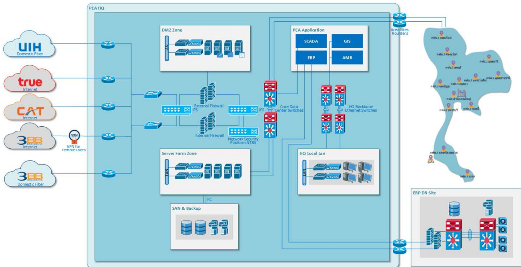
รูปที่ 47 : ภาพแสดงโครงสร้างของระบบเครือข่าย (Network Infrastructure) ของ กฟภ. ในปัจจุบัน
