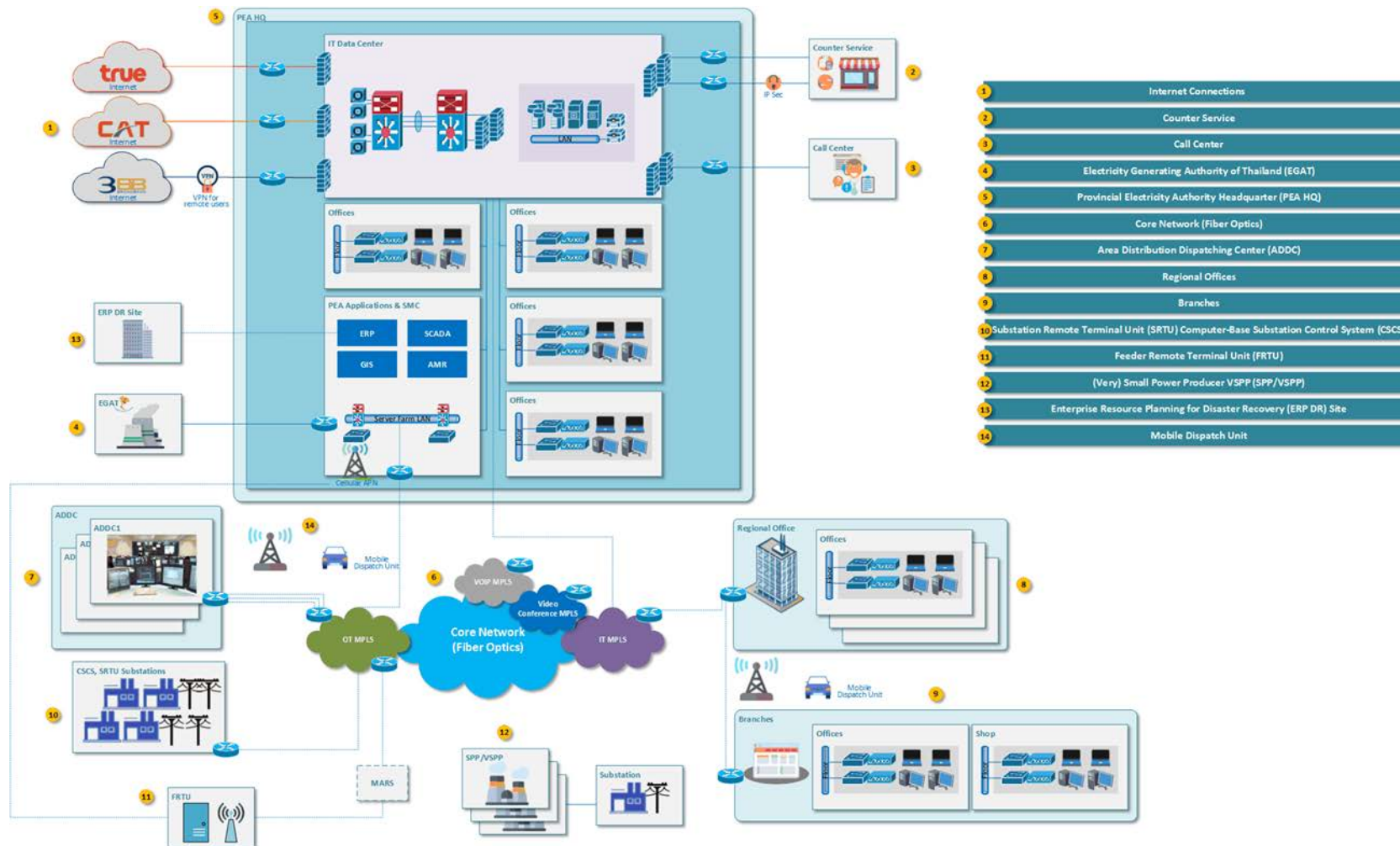
รูปที่ 46 : ภาพแสดงโครงสร้างโดยรวมของระบบเครือข่าย (Environment & Location) ของ กฟภ. ในปัจจุบัน
