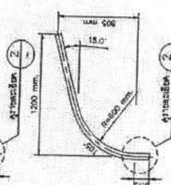
แบบติดตั้งโคมไฟถนน มาตราส่วน 1:75
