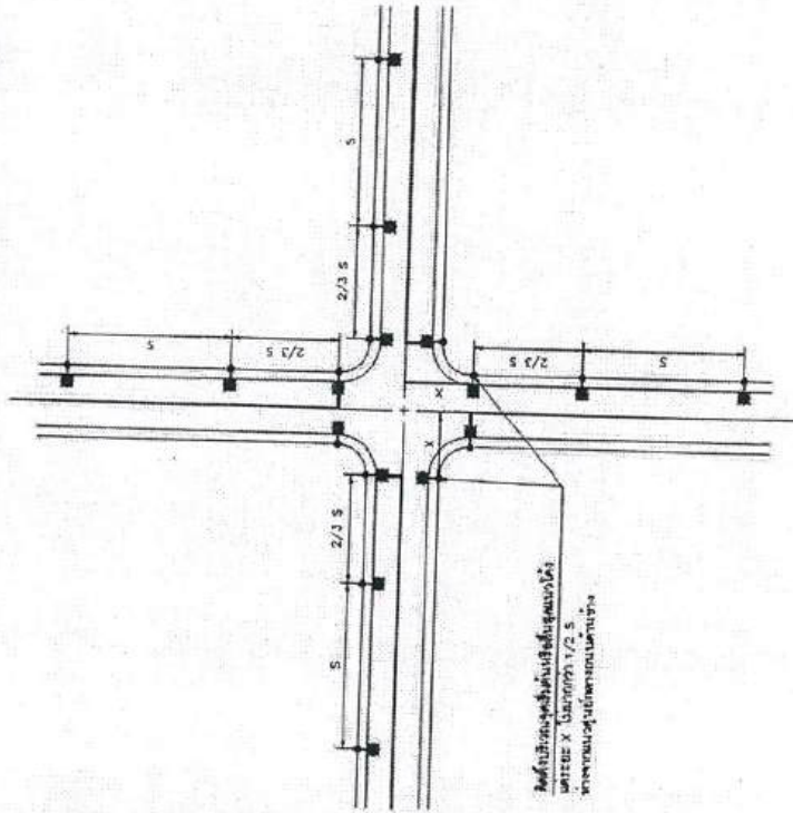
รูปแบบการติดตั้งเสาไฟฟ้าแสงสว่างถนนบริเวณสี่แยก ไม่ลดระดับ
