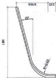
แบบกังไคโมไฟถนน NOT TO SCALE
