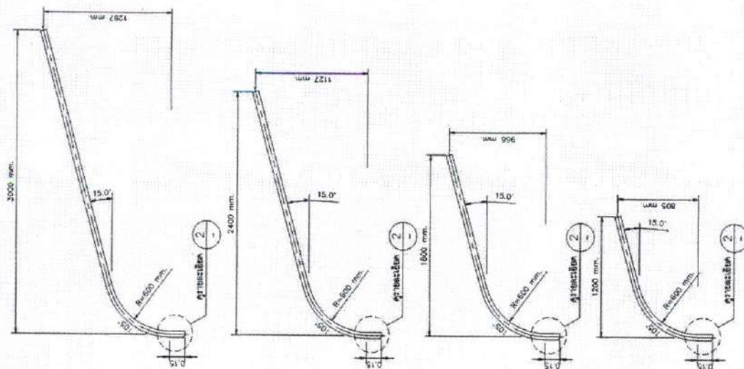
แบบกิ่งคอมไฟถนน ชนิดสวม 1-25
