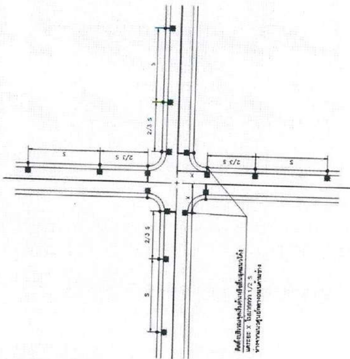
รูปแบบการติดตั้งเสาไฟฟ้าแรงส่งทางถนนบริเวณที่แยก
