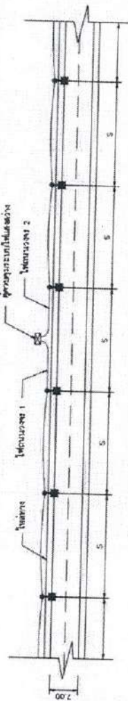
รูปแบบการติดตั้งไฟฟ้าแสงสว่างถนน 2 ช่องทางจราจร บริเวณทางม้าลาย
