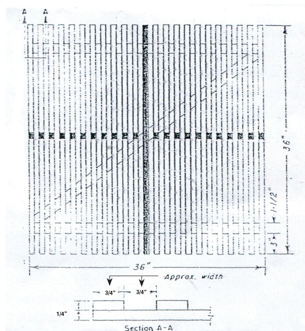
ลักษณะและขนาดของตะแกรงไม้สำหรับสำรวจความชุกของแมลงวัน
