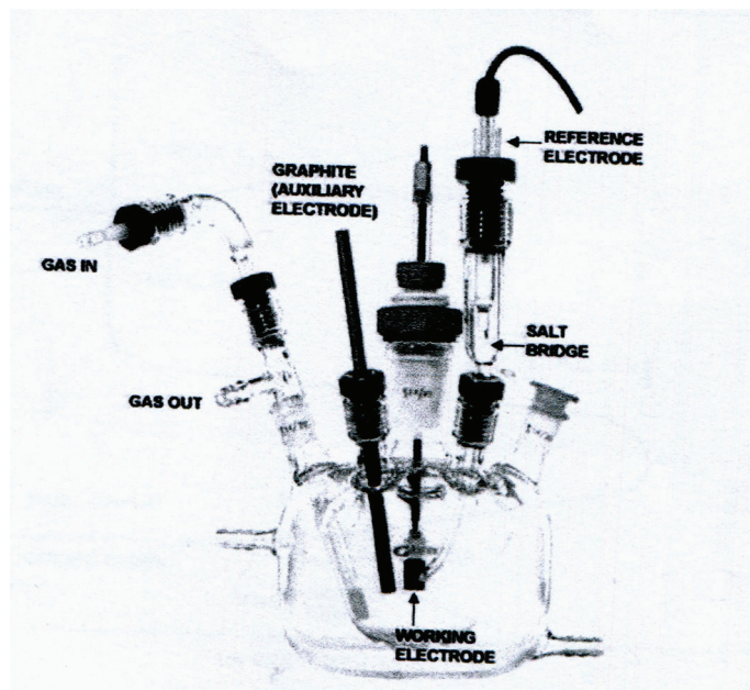
รูปที่ 2-1 แสดงการเตรียมเซลล์ทดสอบ (ข้อ 9.6.4.1)
