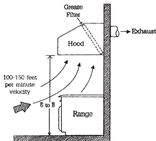
ภาพที่ 1 แสดงการระบายอากาศ โดยพัดลมดูดอากาศ (Hood) บริเวณเหนือเตาไฟ
