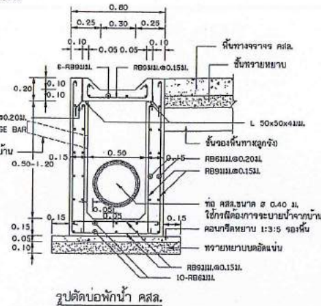
รูปตัดจราจรระบายน้ำ คสล. ในหมู่บ้าน
