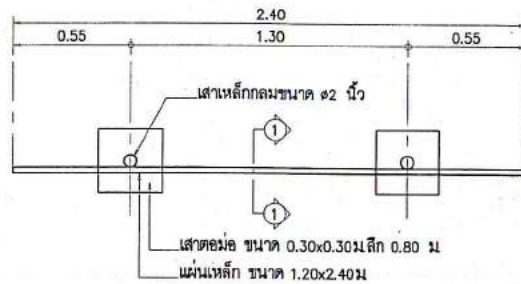
รูปแปลน มาตราส่วน 1 : 25
