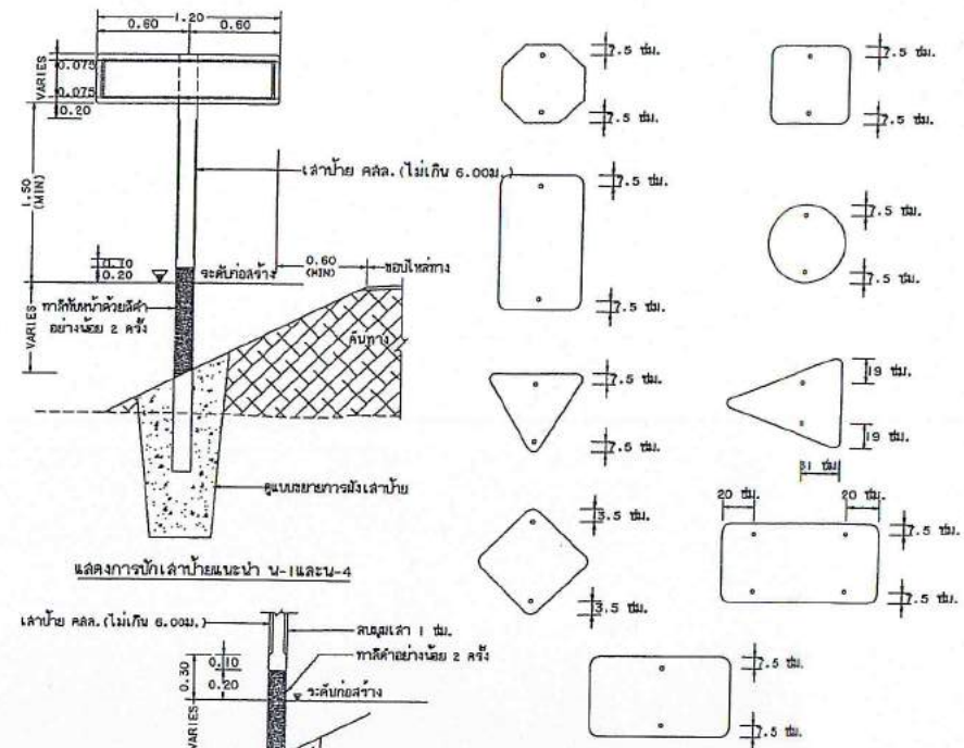
แสดงตำแหน่งการติดตั้งแนบป้ายบังคับ ป้ายเตือน
