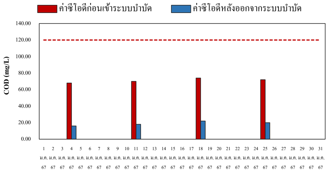
รูปที่ 2-7 กราฟแสดงค่าซีไอดีเปรียบเทียบระหว่าง น้ำก่อนเข้าระบบ และน้ำหลังออกจากระบบบำบัด
