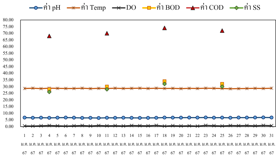
รูปที่ 2-1 กราฟแสดงค่าเฉลี่ยน้ำเสียเข้าสู่ระบบ Headwork
