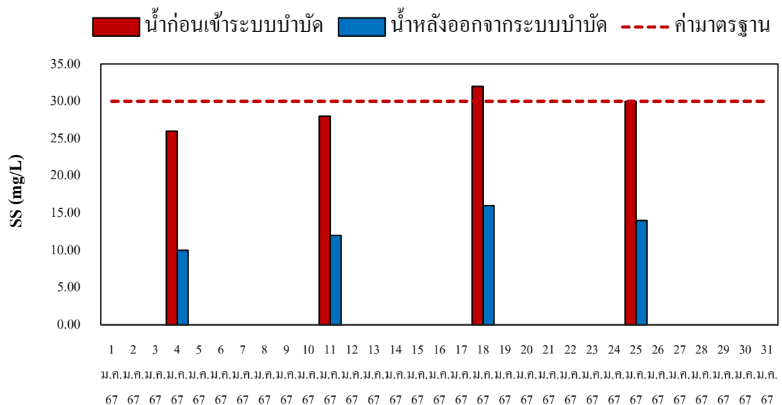
รูปที่ 2-8 กราฟแสดงค่าของแข็งแขวนลอยเปรียบเทียบระหว่าง น้ำก่อนเข้าระบบและน้ำหลังออกจากระบบบำบัด
