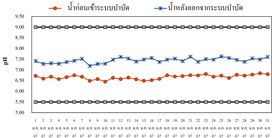
รูปที่ 2-3 กราฟแสดงค่าพีเอช เปรียบเทียบระหว่างน้ำเข้าระบบ และน้ำหลังออกจากระบบบำบัด
