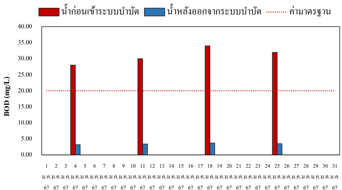
รูปที่ 2-6 กราฟแสดงบีโอดีเปรียบเทียบระหว่าง น้ำเข้าระบบ และน้ำออกจากระบบบำบัด
