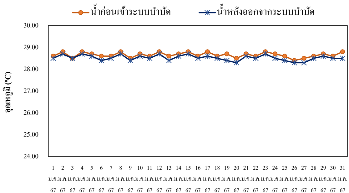
รูปที่ 2-4 กราฟแสดงค่าอุณหภูมิน้ำ เปรียบเทียบระหว่าง น้ำก่อนเข้าระบบ และน้ำออกจากระบบ
