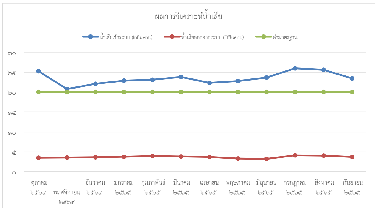
ภาพที่ ๒ แสดงค่า BOD เปรียบเทียบระหว่างน้ำเสียเข้าระบบและน้ำเสียออกจากระบบ
