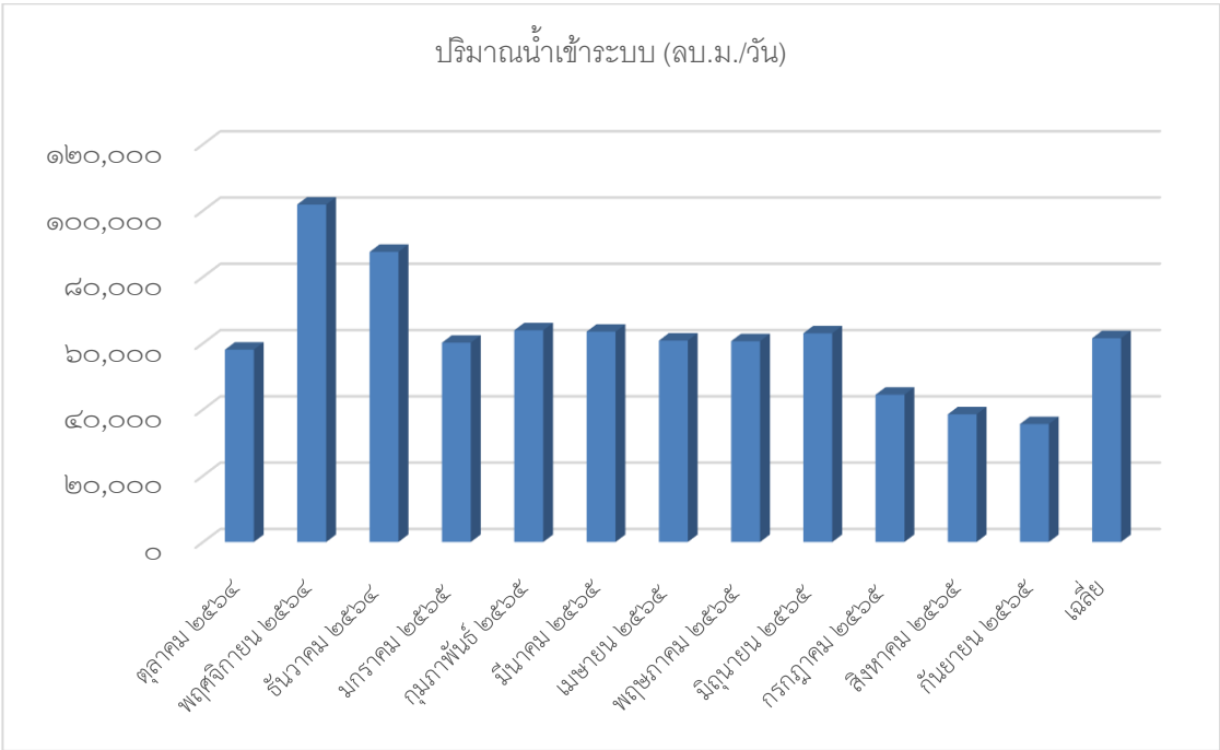
ภาพที่ ๑ แสดงปริมาณน้ำเสียเข้าสู่ระบบบำบัดน้ำเสียเทศบาลนครหาดใหญ่
