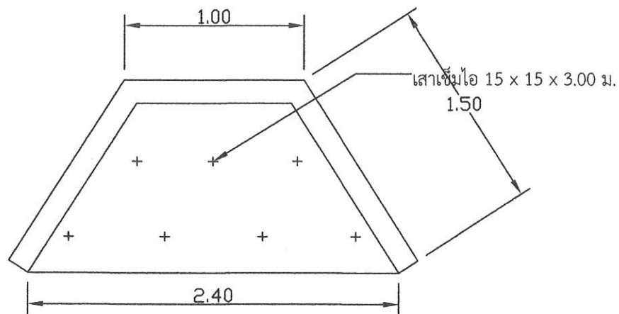
แบบแปลนพื้น
