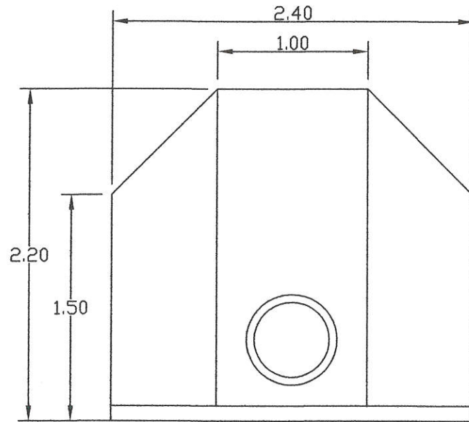
แบบรูปด้านหน้า
