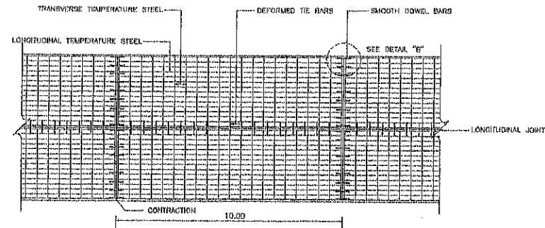
แบบแสดงการเสริมเหล็กถนน ค.ร.ล.
