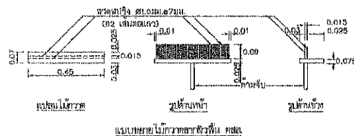
แบบขยายไม้กระดานเสริมพื้น
