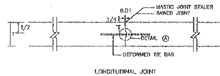
LONGITUDINAL JOINT
