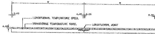
รูปตัดตามขวางของตัวจราจร ค.ร.ล.
